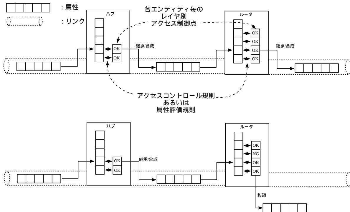
図 4.6: 属性計算の方法
