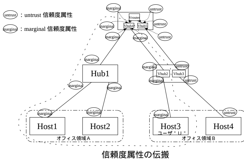
図 5.9: 例題② : 信頼度属性の伝搬の分離
