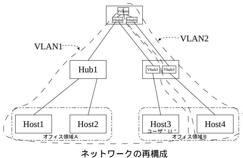
図 5.8: 例題② : ネットワークの再構成
