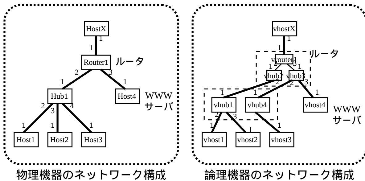
図 5.1: ネットワーク構成記述例 (物理構成と論理構成)
