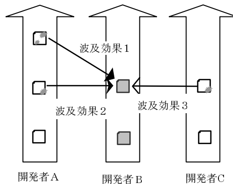
図 3.7: 競合の検知
