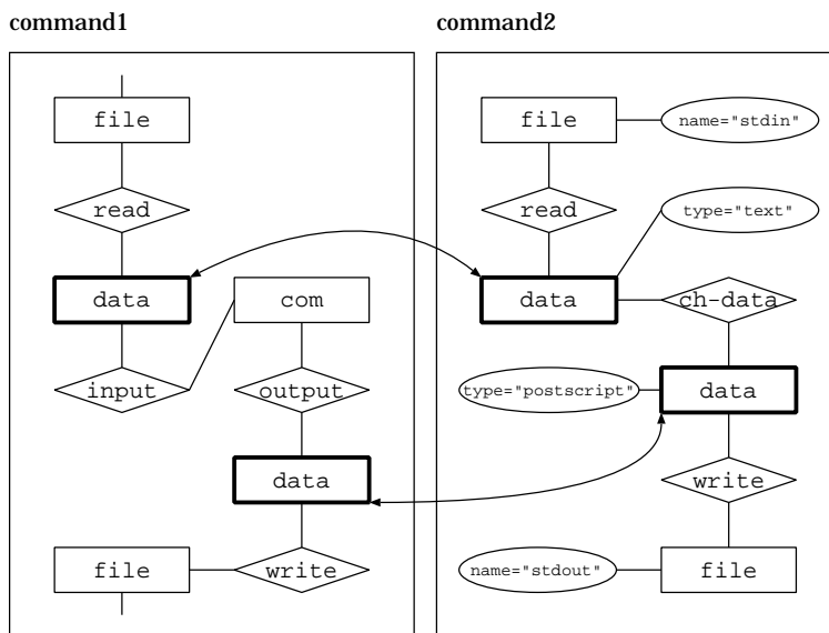
図 4.1 3: command型の変換の例 (変換前)
