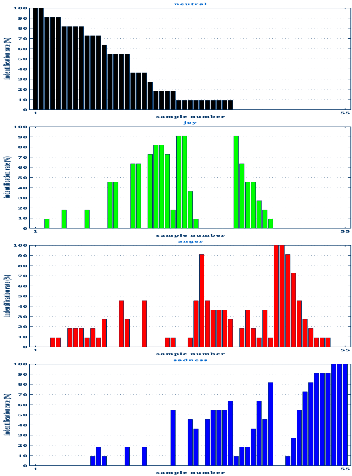
図 2.2: 感情分類実験の結果
