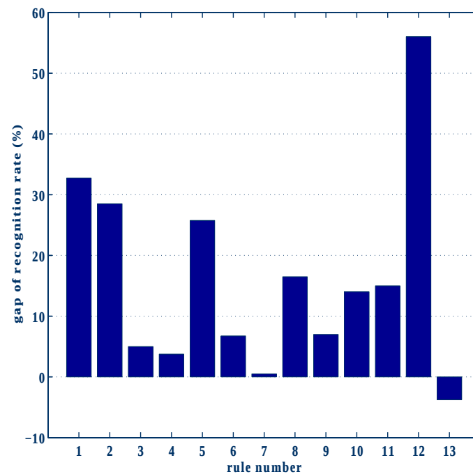
図 6.5: 物理量変換ルールによる認識率の向上
