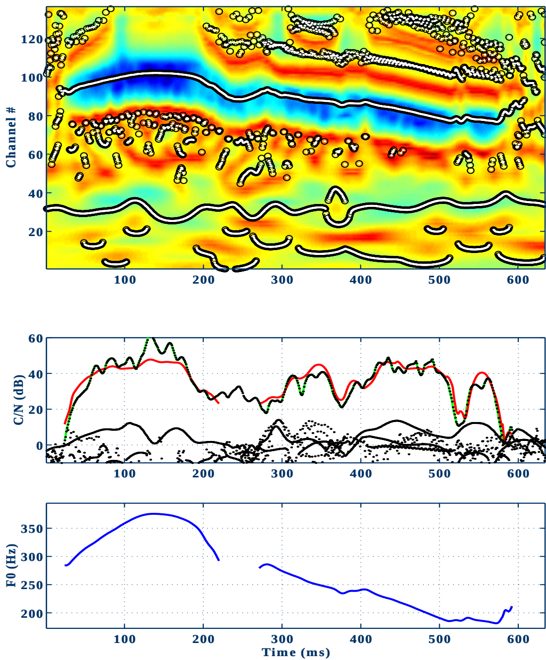
図 3.1: TEMPO2 による基本周波数推定結果
