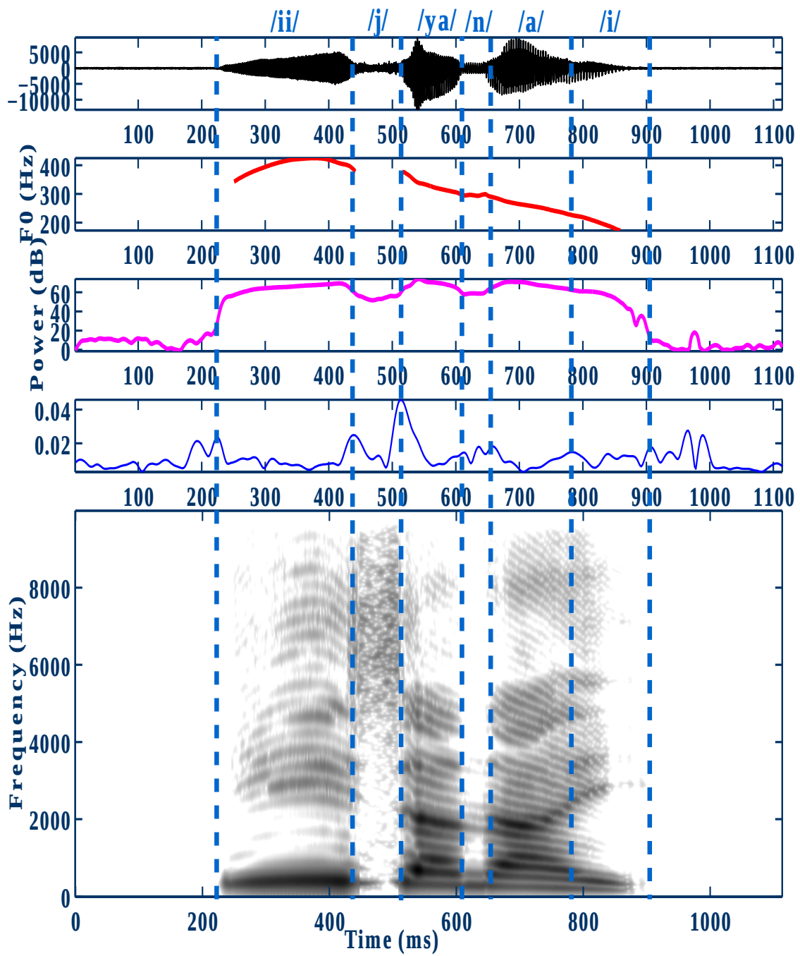
図 4.1: 時間変化パターンの抽出結果
