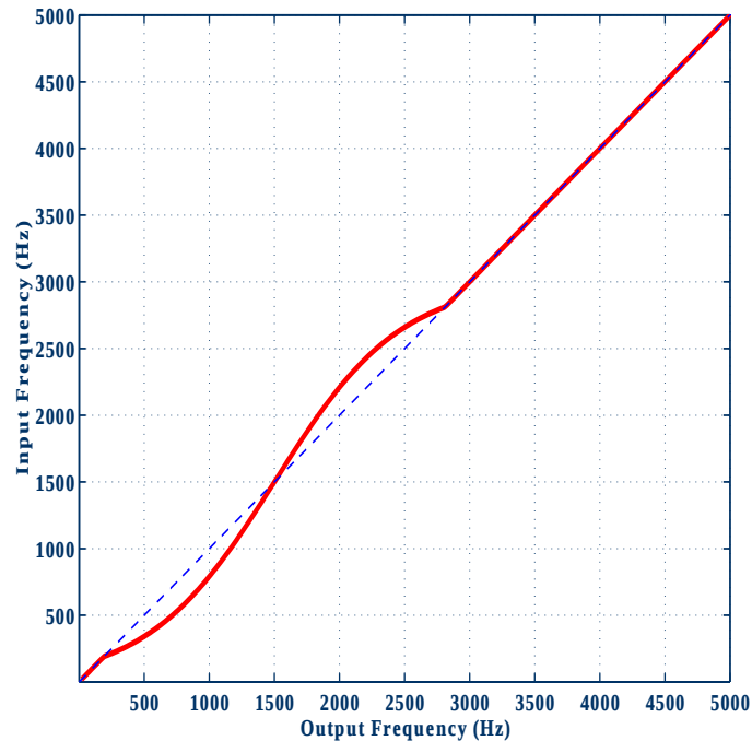
図 5.4: ホルマント周波数のシフト
