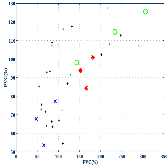
図 4.7: 分析結果 - 音韻/ai/でのパワー・基本周波数の変化率
