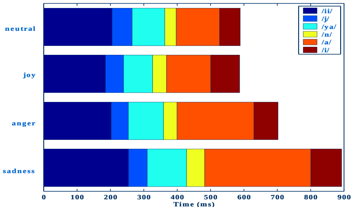
図 5.1: 音韻毎の発話時間
