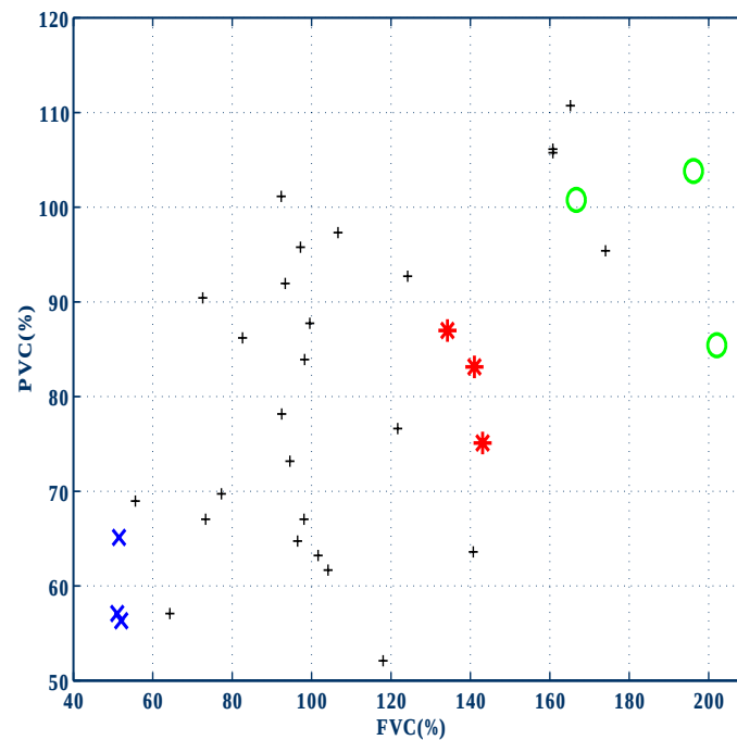
図 4.3: 分析結果 - 全発声区間での基本周波数・パワーの変化率
