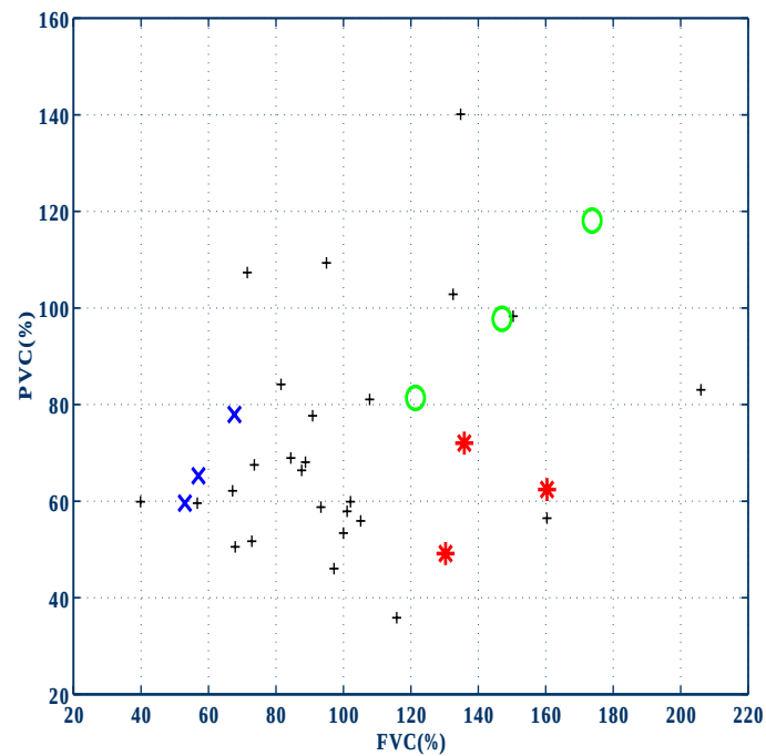
図 4.6: 分析結果 - 音韻/ii/でのパワー・基本周波数の変化率
