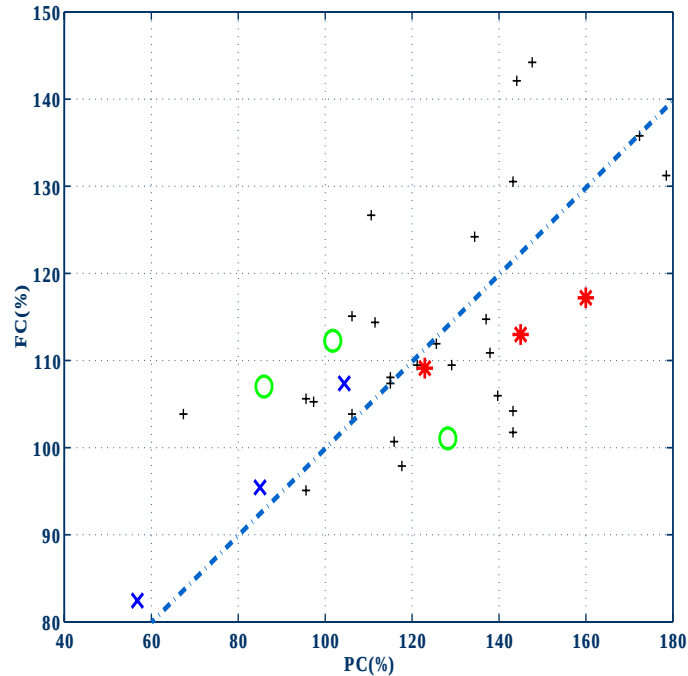
図 5.3: パワーと基本周波数の関係
