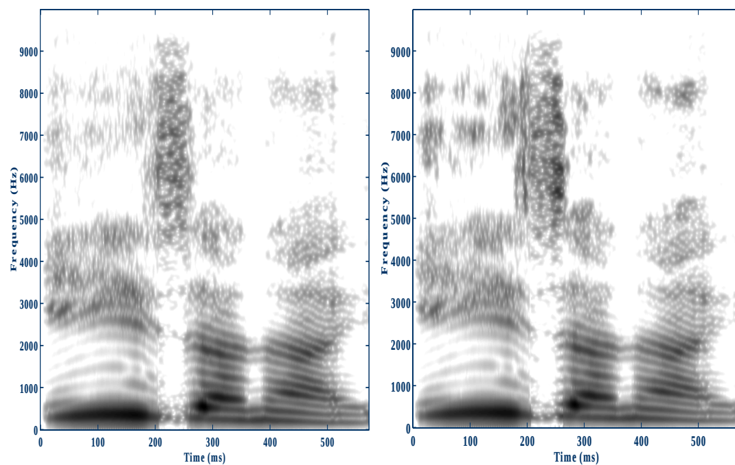
図 5.5: 高域スペクトル成分の増加
