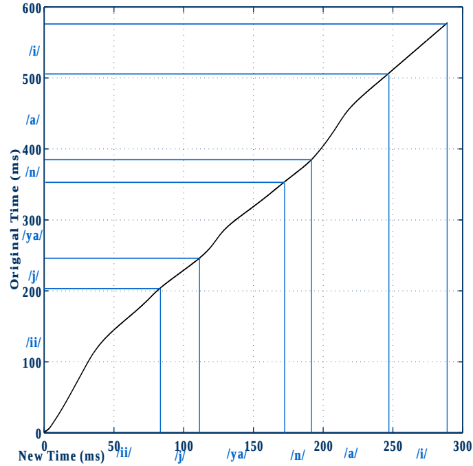
図 5.2: 発話時間の伸縮
