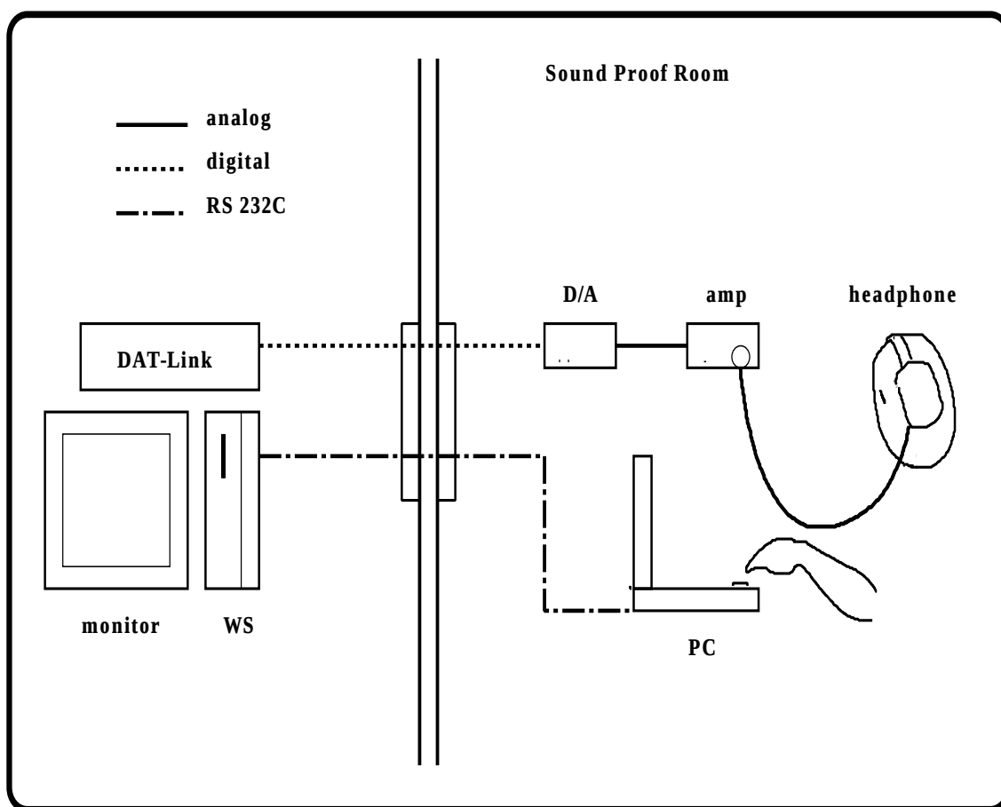
図 2.1: 実験システム
