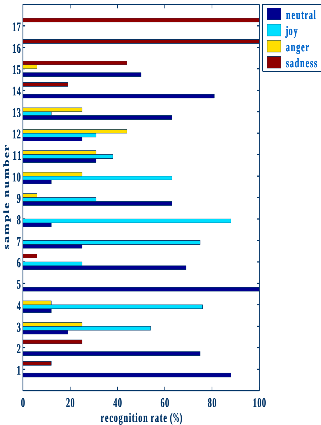
図 6.4: 実験結果 - 「もちろん発表のときも日本語でよろしいですね」
