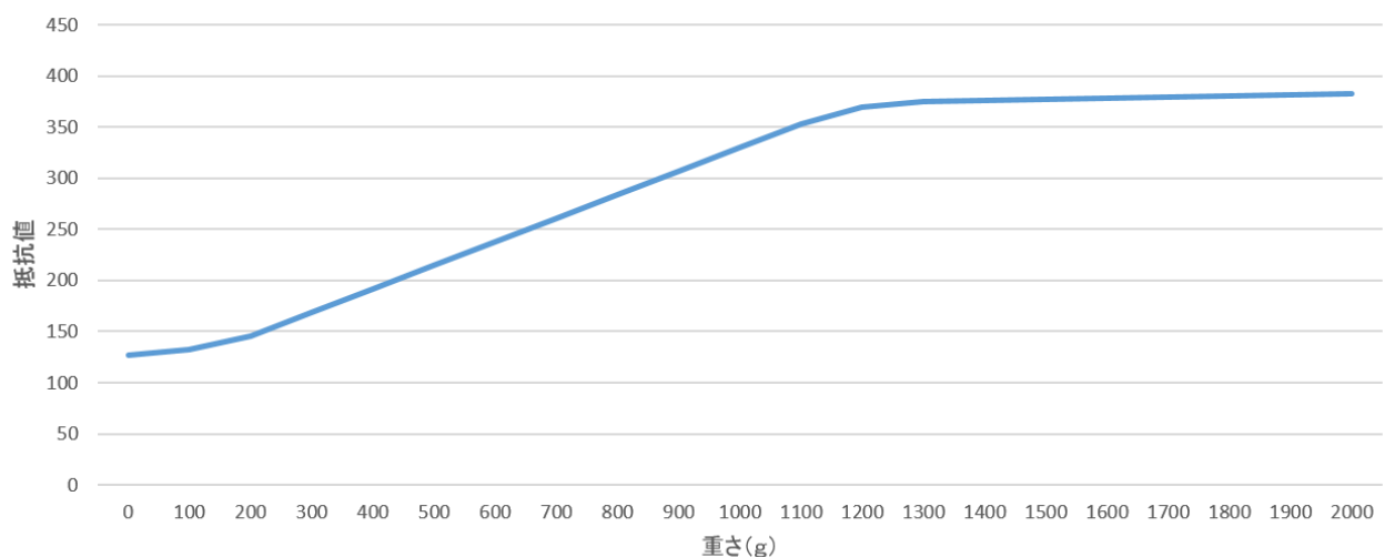
Figure19 抵抗値と重量のマッピング
