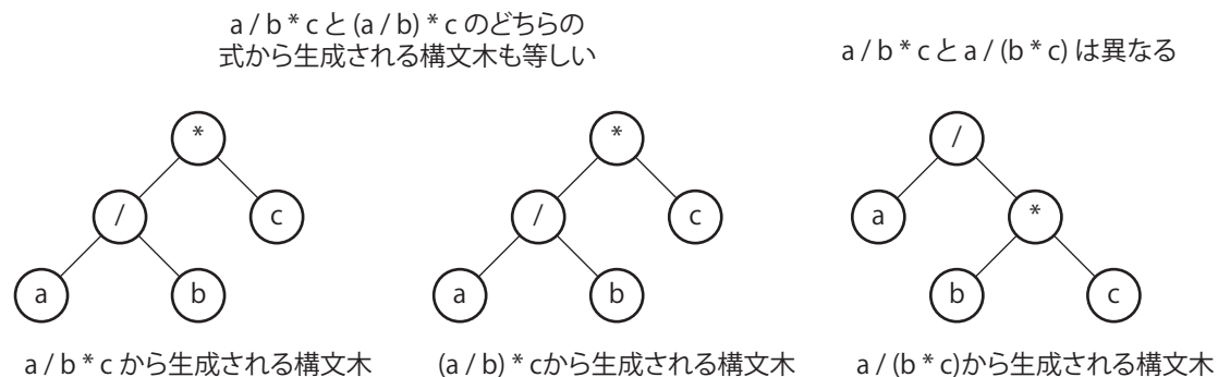
図 3.7: コンパイラの LR 構文解析の例
