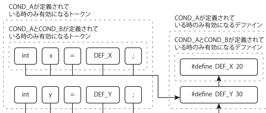
図 3.3: プリプロセッサ情報付きトークン列を作成する例
