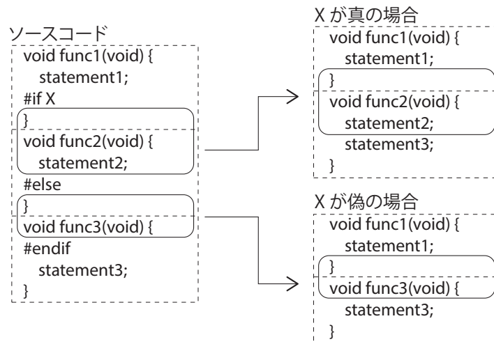
図 3.1: 構文解析が困難であるソースコードの例
