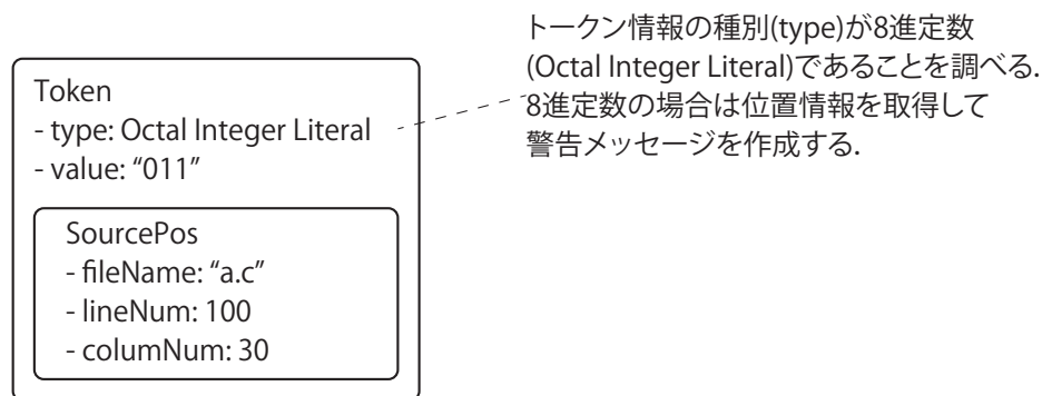
図 3.9: 8進定数を検出する例
