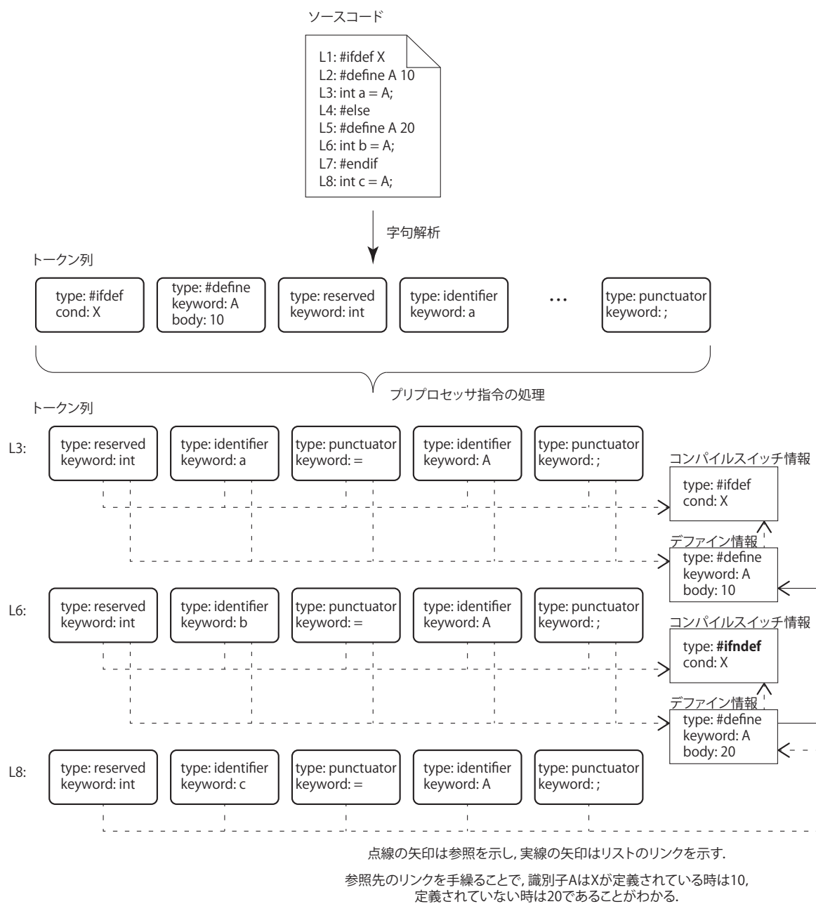
図 3.5: プリプロセッサ指令の処理の例
