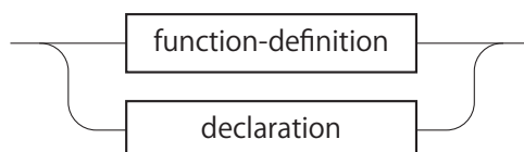
図 A.58: external-declaration
