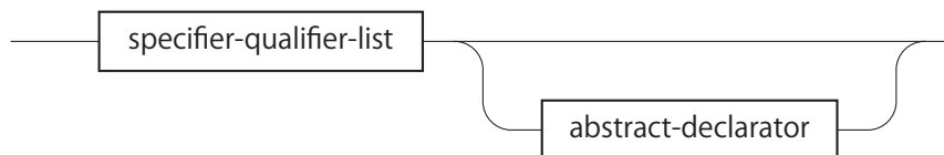
図 A.38: type-name
