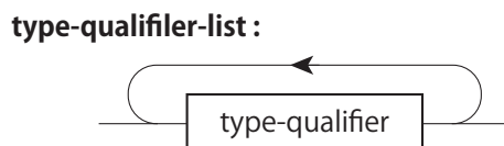
図 A.34: type-qualifier-list
