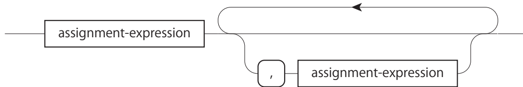
図 A.3: argument-expression-list
