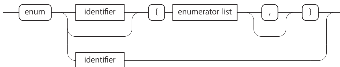
図 A.25: enum-specifier
