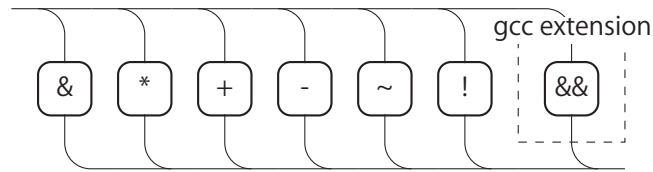
図 A.5: cast-expression
