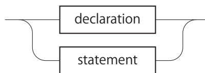
図 A.52: block-item
