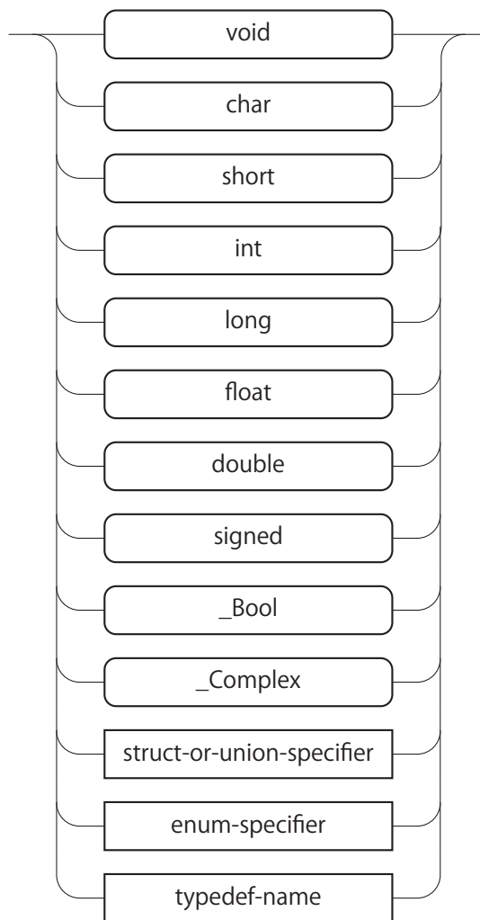
図 A.17: type-specifier
