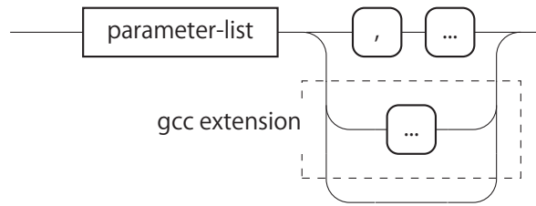
図 A.35: parameter-type-list
