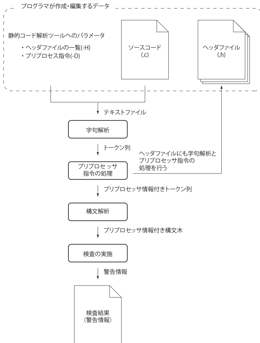
図 3.4: 本研究で作成した静的解析ツールの処理の流れ
