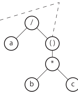
a / (b * c) から生成される構文木
