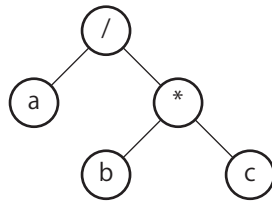
a / b * c から生成される構文木
