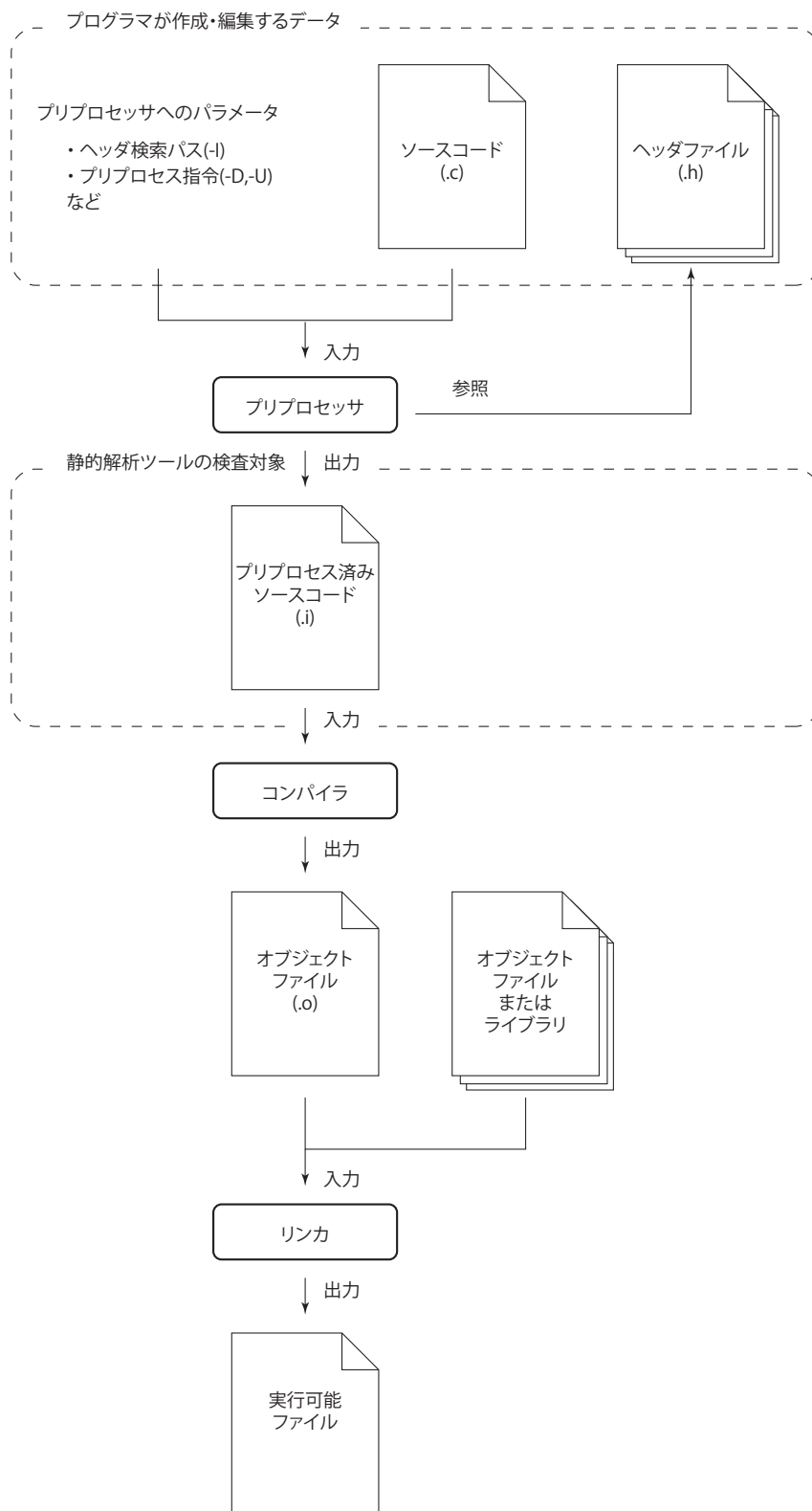
図 3.2: プリプロセッサ, コンパイラ, リンカの処理の流れ
