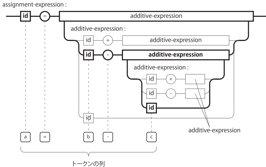
図 3.6: 単純なパーサの例
