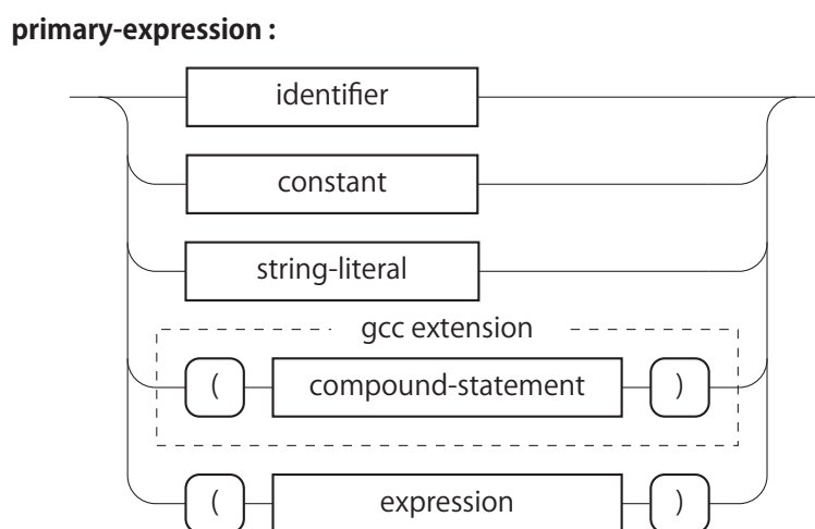
図 A.1: primary-expression
