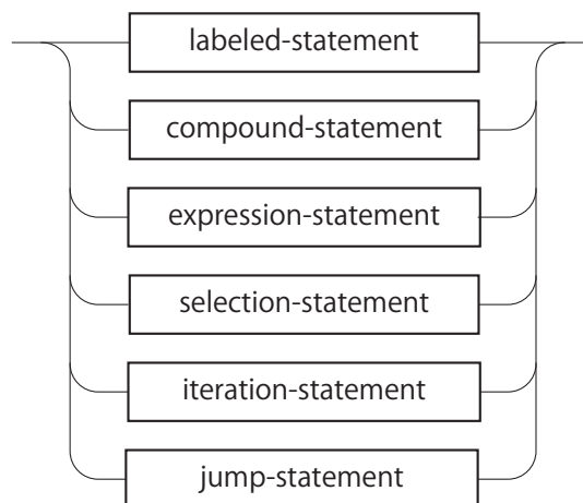
図 A.48: statement
