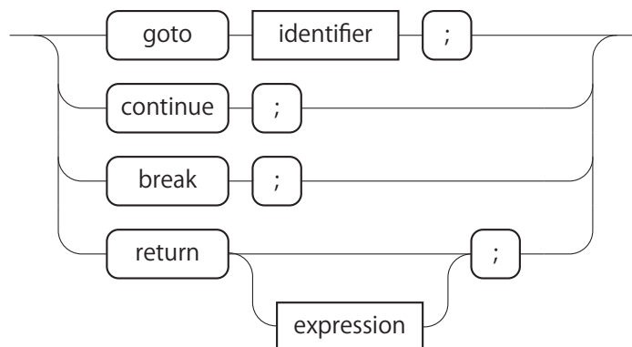
図 A.56: jump-statement
