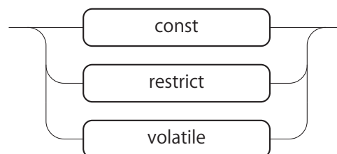
図 A.28: type-qualifier
