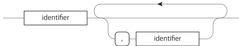
図 A.37: identifier-list
