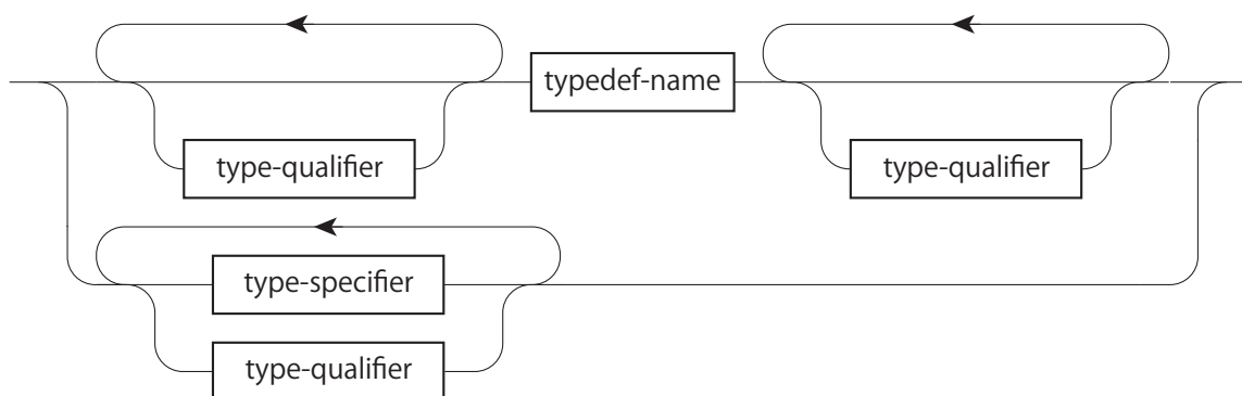
図 A.22: specifier-qualifier-list
