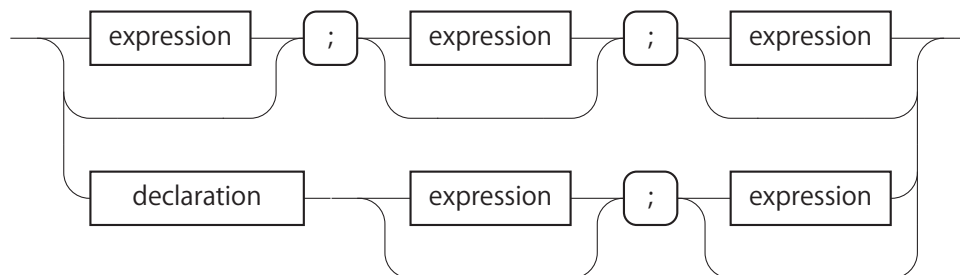
図 A.55: iteration-statement
