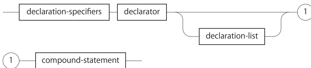
図 A.59: function-definition
