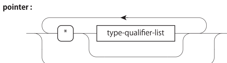
図 A.33: pointer
