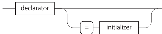
図 A.15: init-declarator-list
