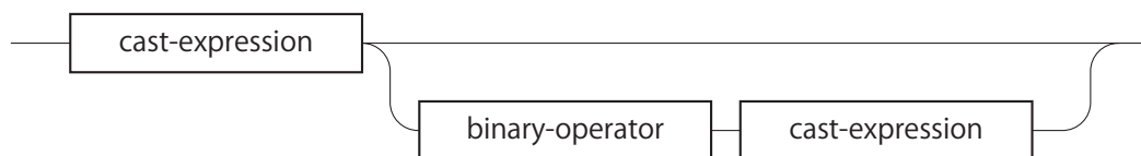
図 A.7: binary-operation-expression
