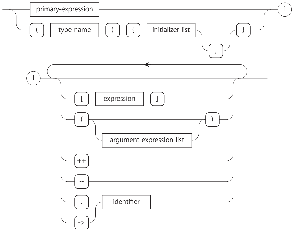
図 A.2: postfix-expression
