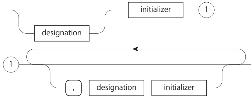
図 A.43: initializer-list
