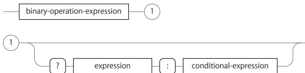
図 A.8: conditional-expression
