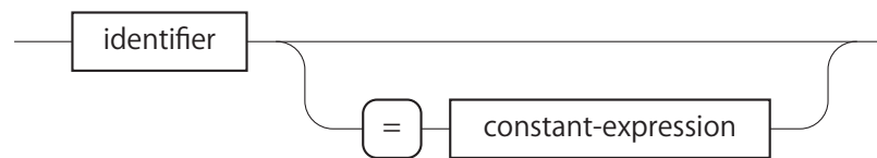
図 A.27: enumerator
