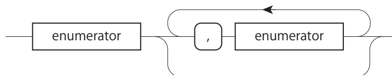
図 A.26: enumerator-list
