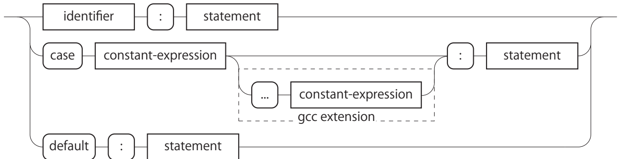
図 A.49: labeled-statement
