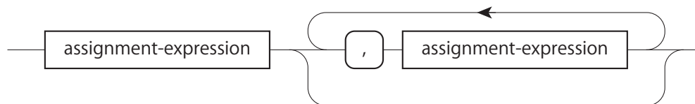
図 A.10: expression
