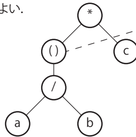
(a / b) * c から生成される構文木
