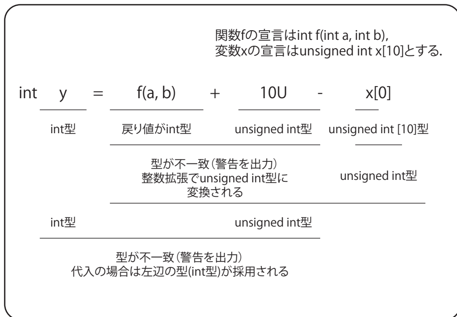
図 3.10: 型の不一致を検出する例 (マクロなし)
