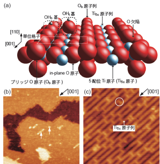
図1 (a) TiO_2 (110)-(1×1)表面のモデル図。赤色の大円、青色の小円、灰色の大円は、それぞれO原子、Ti原子、H原子を表す。(b)(c) TiO_2 (110)-(1×1)表面のSTM像。(b): 40 \times 40 \text{ nm}^2 , (c): 10 \times 10 \text{ nm}^2 。試料バイアス ( V_s ): +1.4 V、トンネル電流 ( I_t ): 0.2 nA。
