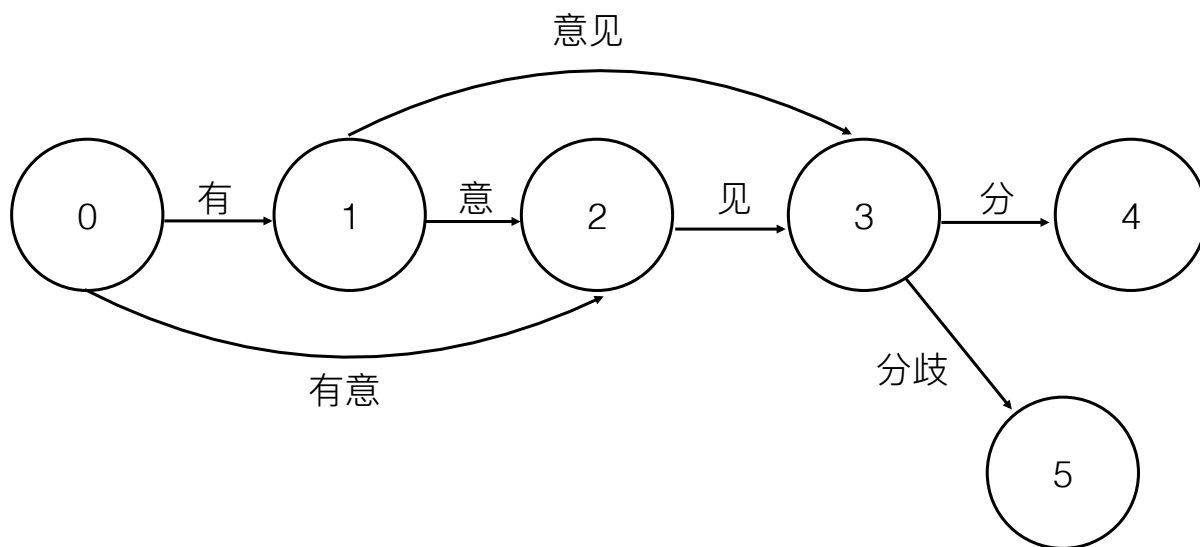
図 2.1: DAG の例
