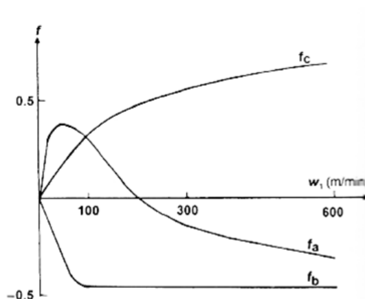
Figure 4-5 巻き取り速度による結晶配向度の変化 27)
