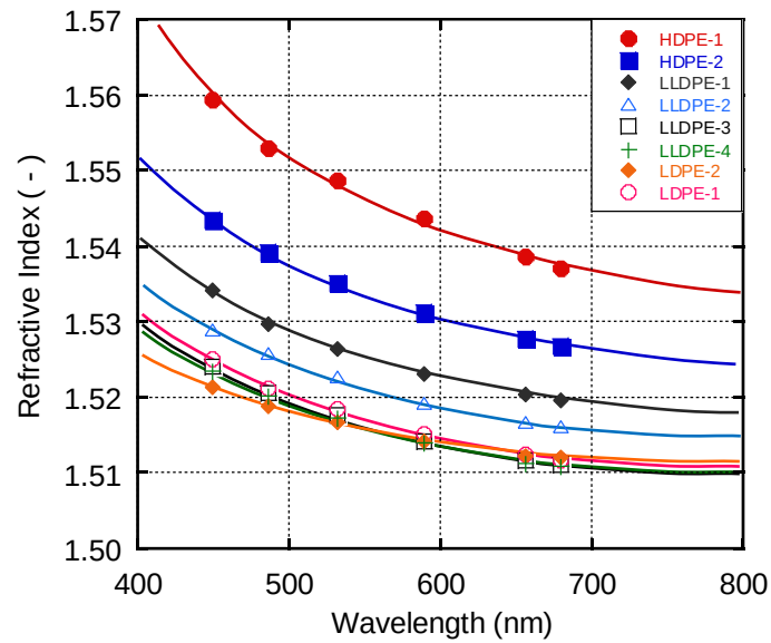
Figure 4-15 屈折率の波長依存性
