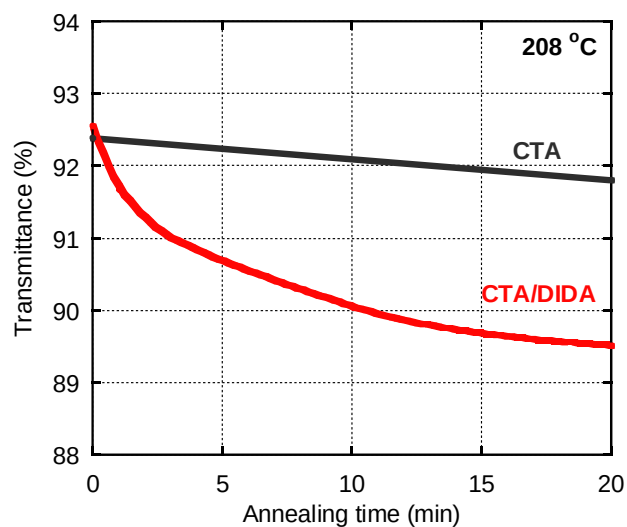
Figure 3-14 加熱に伴う全光線透過率の変化
