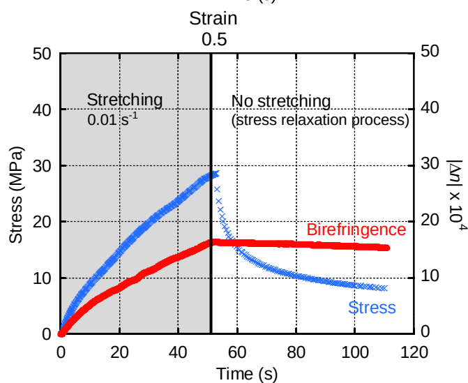
Figure 2-12 加熱一軸延伸における応力－光学同時測定
