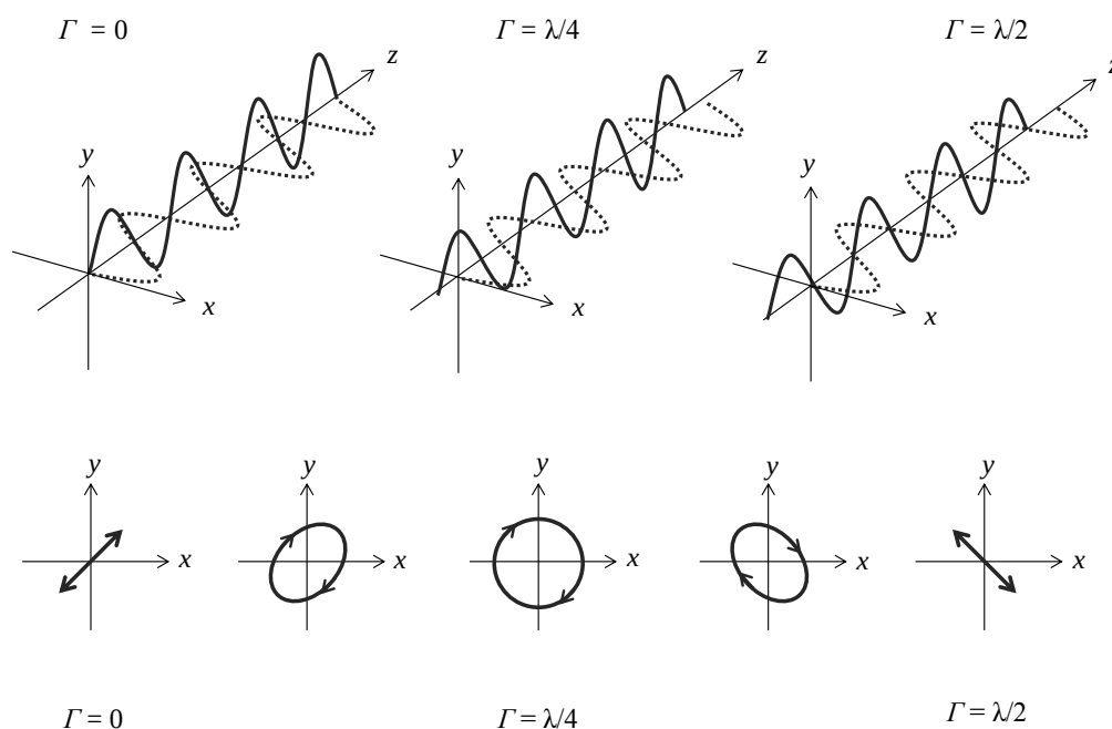
Figure 3-1 位相差と偏光状態
