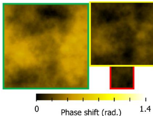
図1 真空領域において 322 \times 322 , 241 \times 241 , 83 \times 83 \text{ nm}^2 の領域から得られた3枚の位相像を示す。
