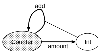
図 2.1: モジュール Counter の ADJ 図
