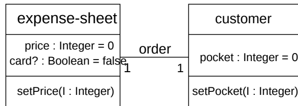
図 4.3: クラス図: シミュレーション実行例 (1)
