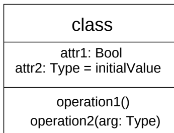
図 3.4: クラス図
