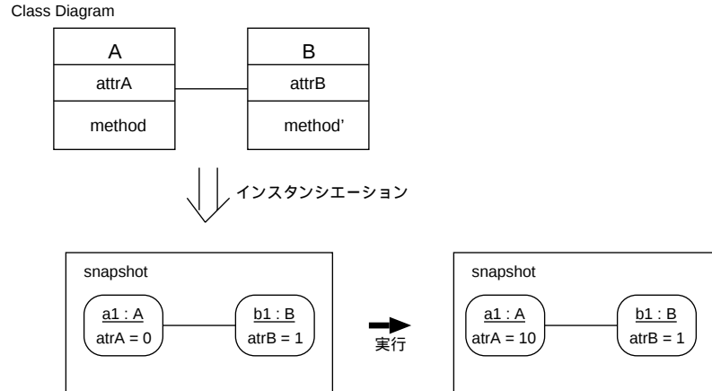
図 4.1: シミュレーション実行
