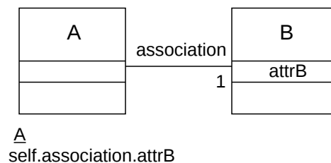
図 3.7: 多重度 1 の場合の関連による誘導
