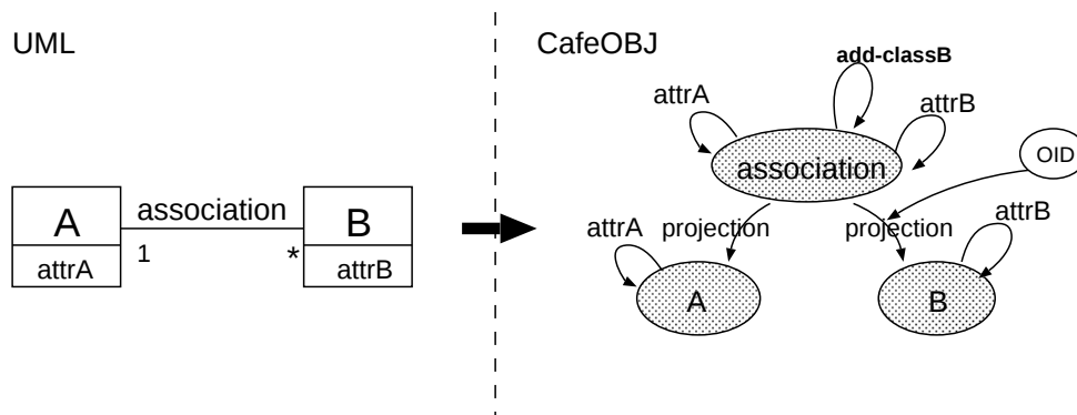
図 3.6: 多重度付き関連の扱い
