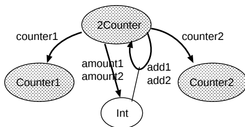
図 2.2: モジュール 2COUNTER の ADJ 図
