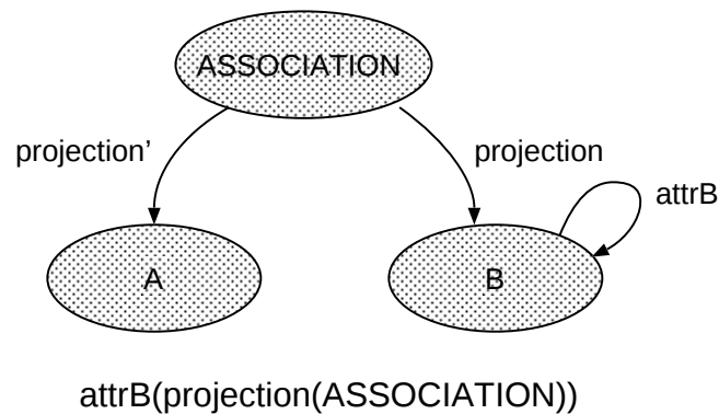
図 3.9: 多重度 1 の場合の関連による誘導の振舞仕様による扱い
