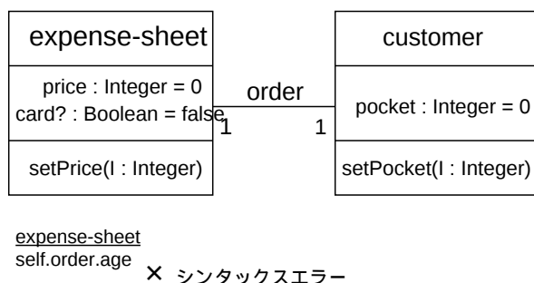
図 4.5: Type チェックのイメージ
