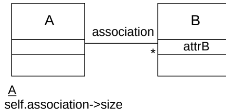
図 3.8: 多重度 1 以上の場合の関連によるコレクション型
