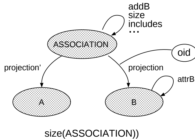
図 3.10: 多重度 1 以上の場合の関連によるコレクション型の振舞仕様による扱い
