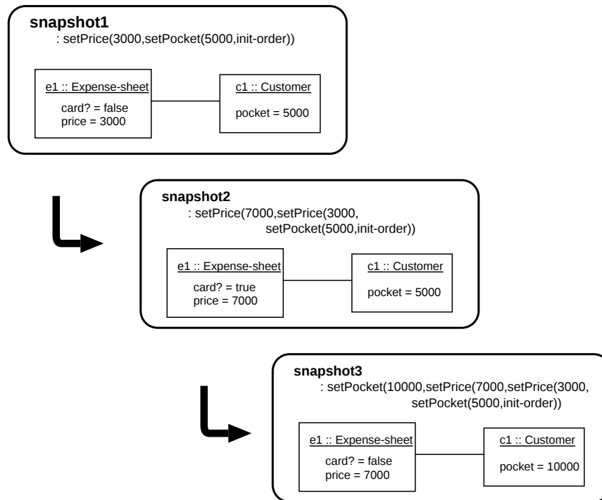
図 4.4: シミュレーション実行例 (1)
