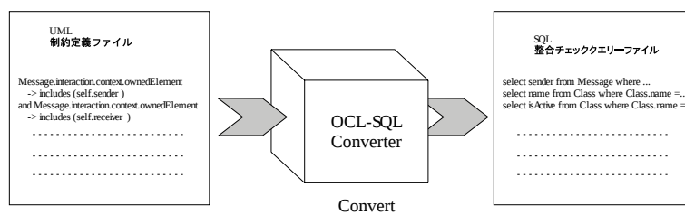
図 2.6: OCL-SQL Converter
