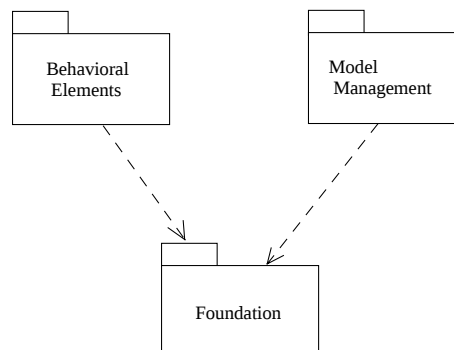
図 3.2: トップレベルパッケージ
