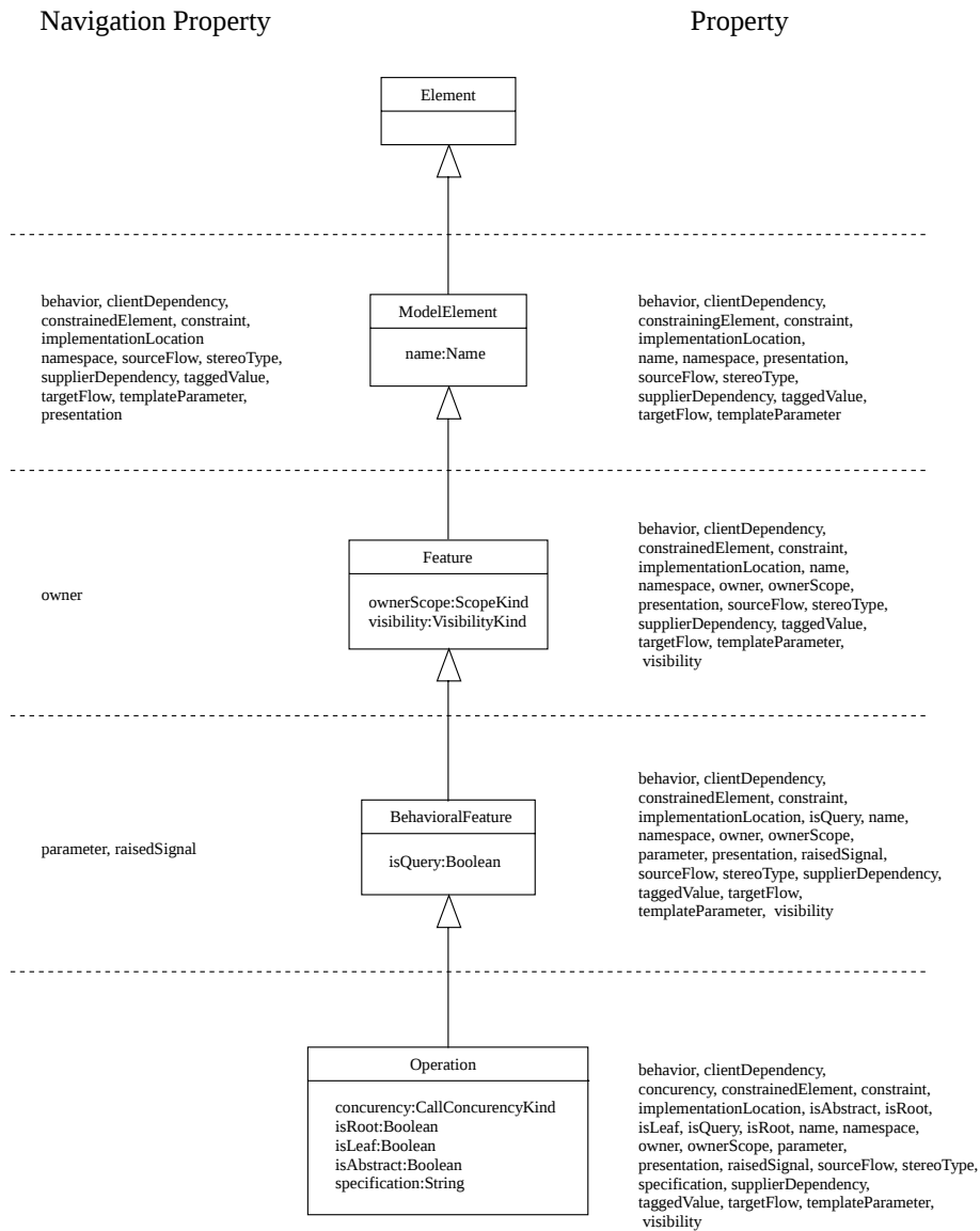
図 5.17: “Operation” までのプロパティの継承
