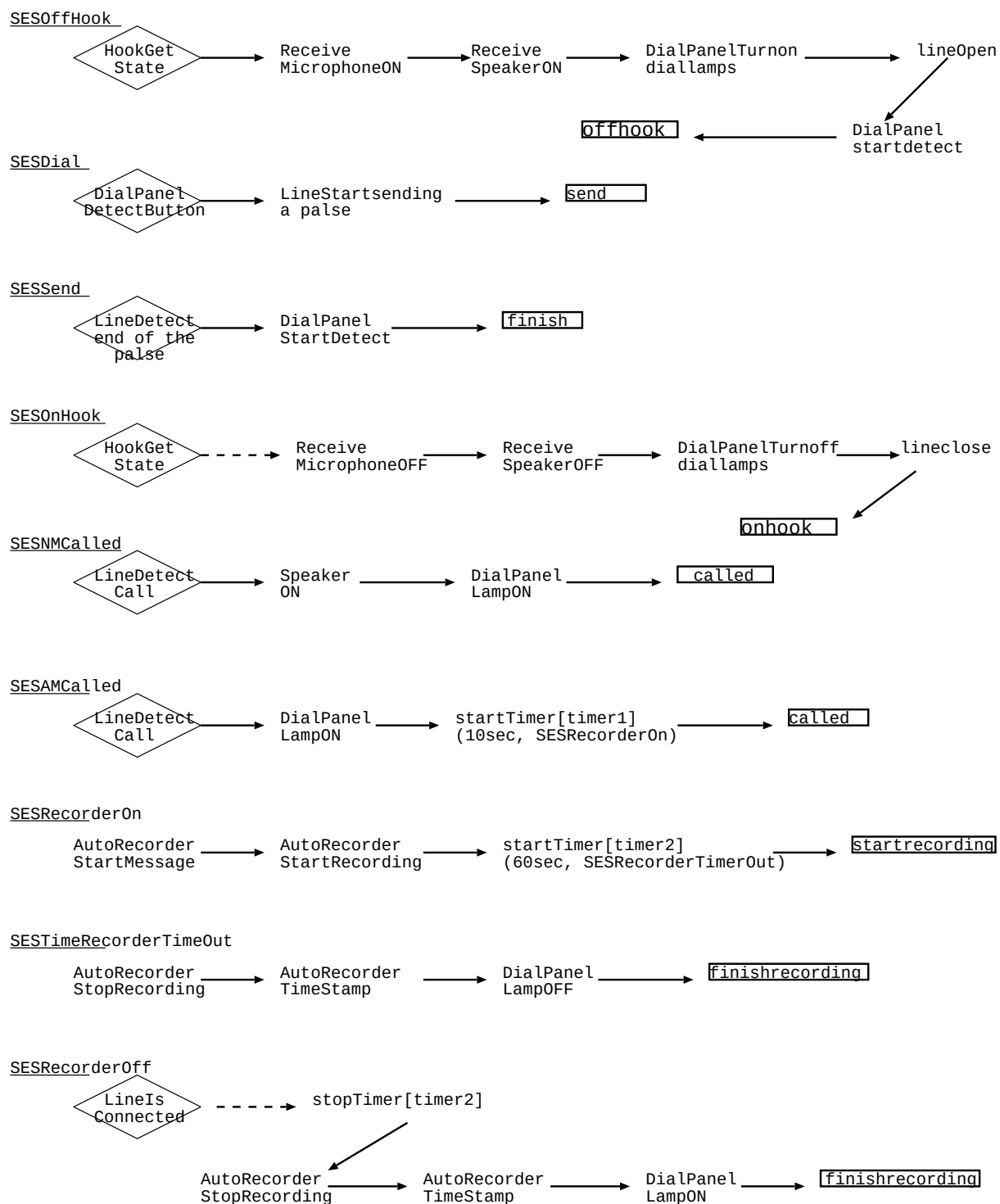
図 4.2: SES の定義
