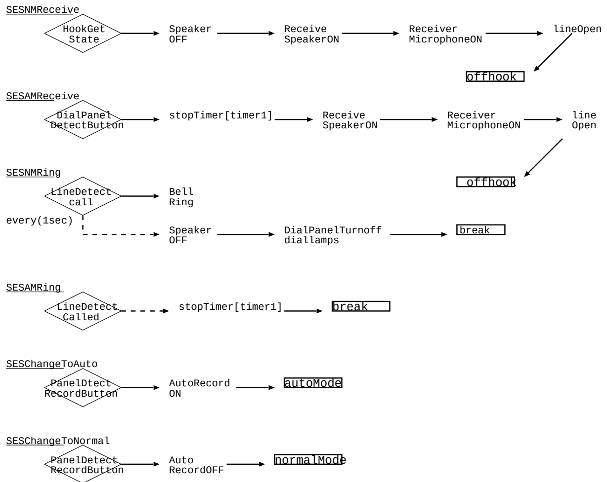
図 4.3: SES の定義
