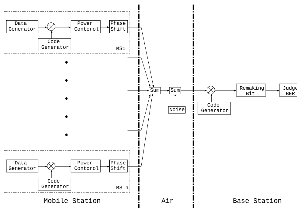
図 6.3: チャンネル多重化のシミュレーションモデル
