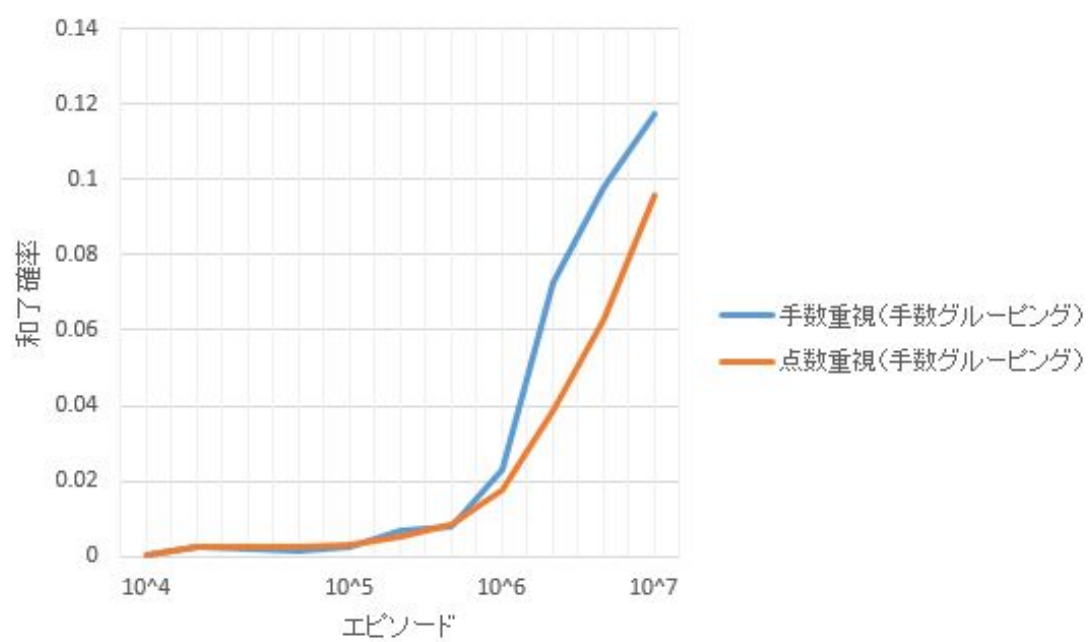
図 6.6: 手数グルーピング和了確率
