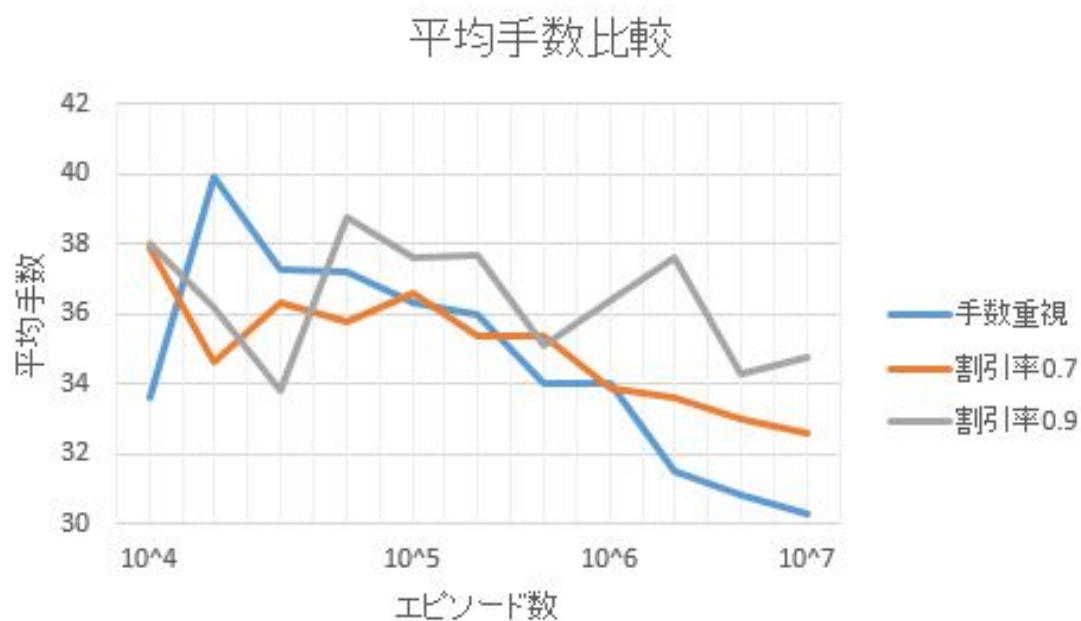
図 6.1: 平均手数の比較
