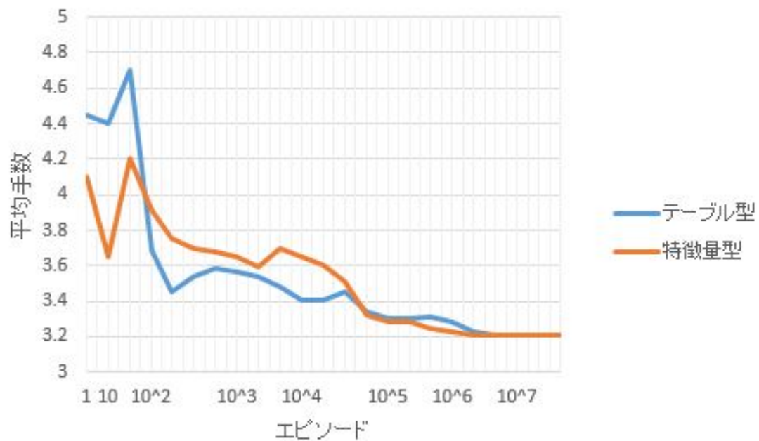
図 5.2: テーブル型と特徴量型の学習時曲線
