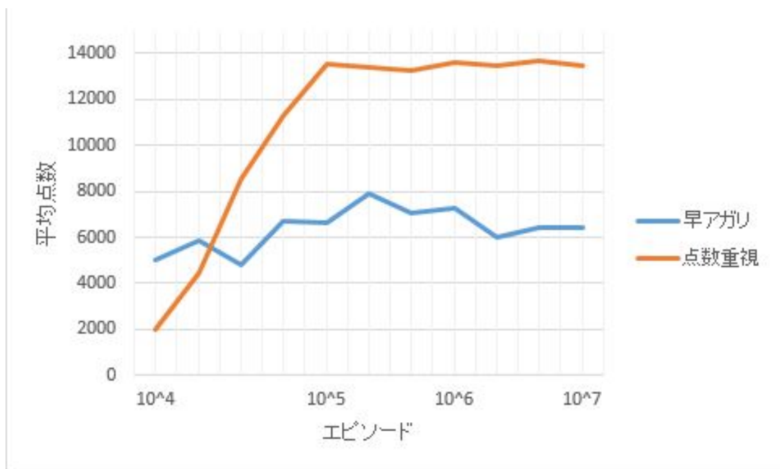
図 5.7: 平均点数の比較
