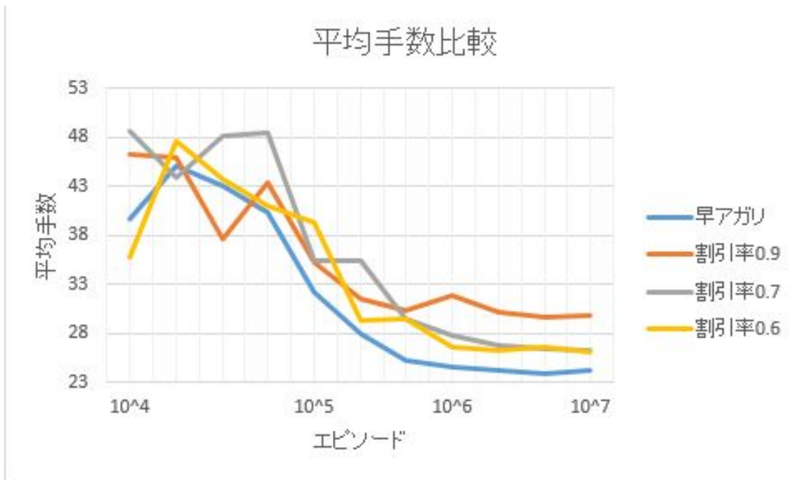
図 5.8: 平均手数の比較
