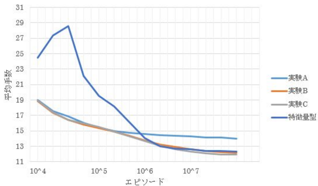
図 5.4: 2 色 5 枚麻雀の平均手数の比較
