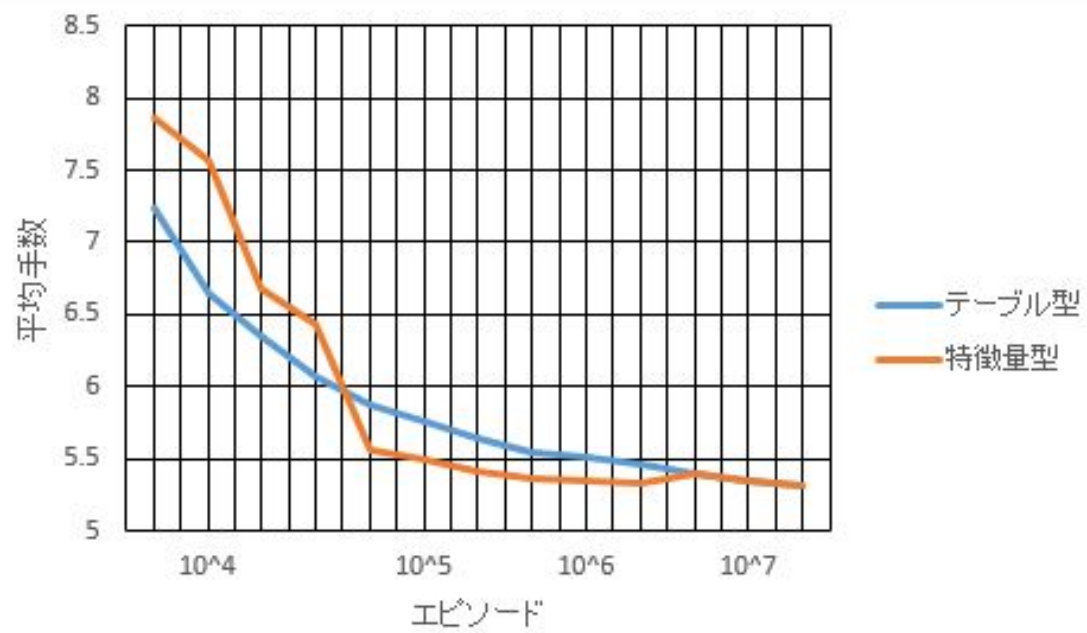
図 5.3: 1 色 5 枚麻雀の平均手数の推移
