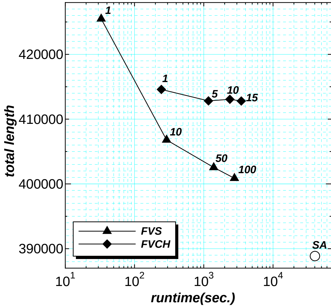
図 3.14: data100 に対するフォース値に基づく手法での総配線長と実行時間の関係（各点に付された数は#loops を表す）
