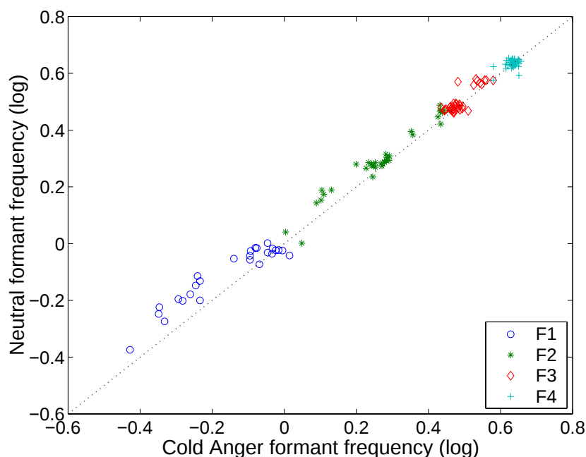
図 1: 「Neutral」と「Cold Anger」のフォルマント周波数の関係
