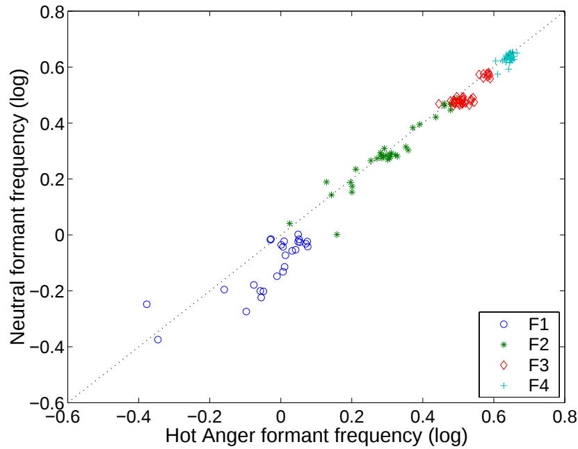
図 2: 「Neutral」と「Hot Anger」のフォルマント周波数の関係
