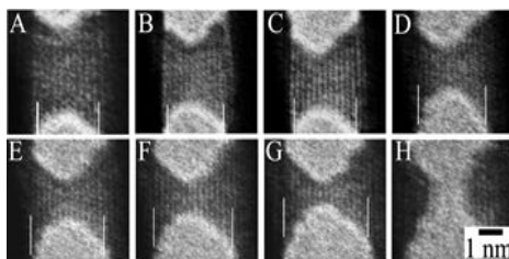
図(2) 金[111]接点の TEM 像. 金接点を引っ張り(A-G)、切断した(H)。
