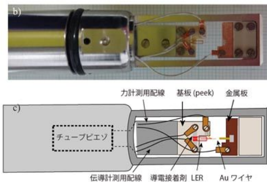
図(7) 開発した TEM-AFM ホルダーの写真と模式図
