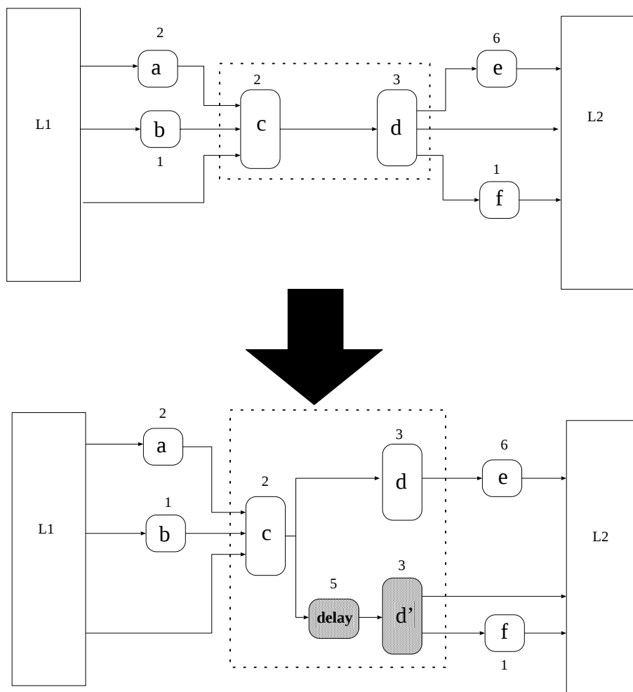
図 4.4: 遅延挿入に伴う回路の冗長化
