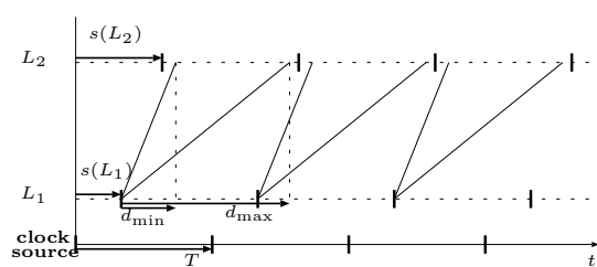
図 3.1: パイプラインと遅延
