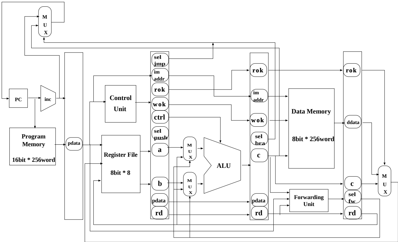
图 5.1: WAVIST 概略回路图
