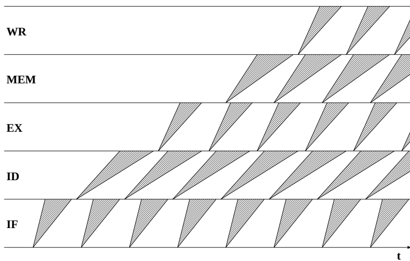
図 2.2: ウェーブパイプライン回路
