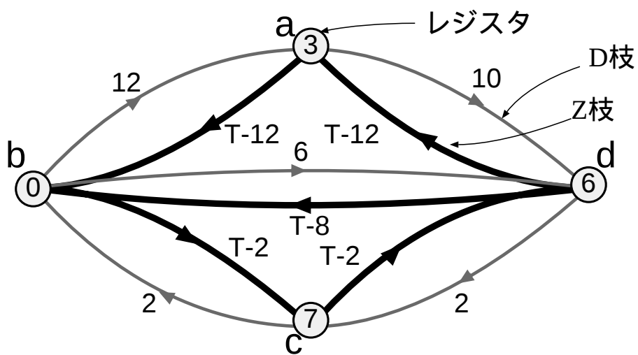
図 2.6: 制約グラフ
