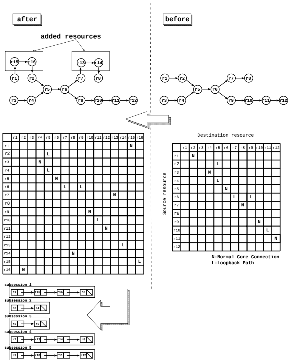
図 5.9: セッション分解法
