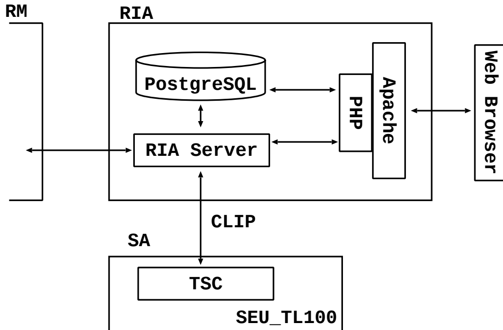
図 8.4: リソースインフォメーションエージェントの実装
