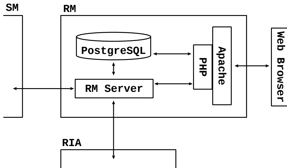
図 8.5: リソースマネージャの実装
