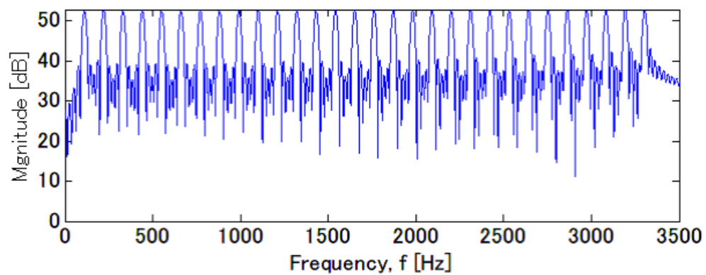
図 5.3: 時変調波複合音の調波構造
