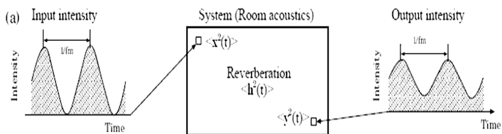
図 4.7: 残響が AM 成分に与える影響 (鵜木) [72]
