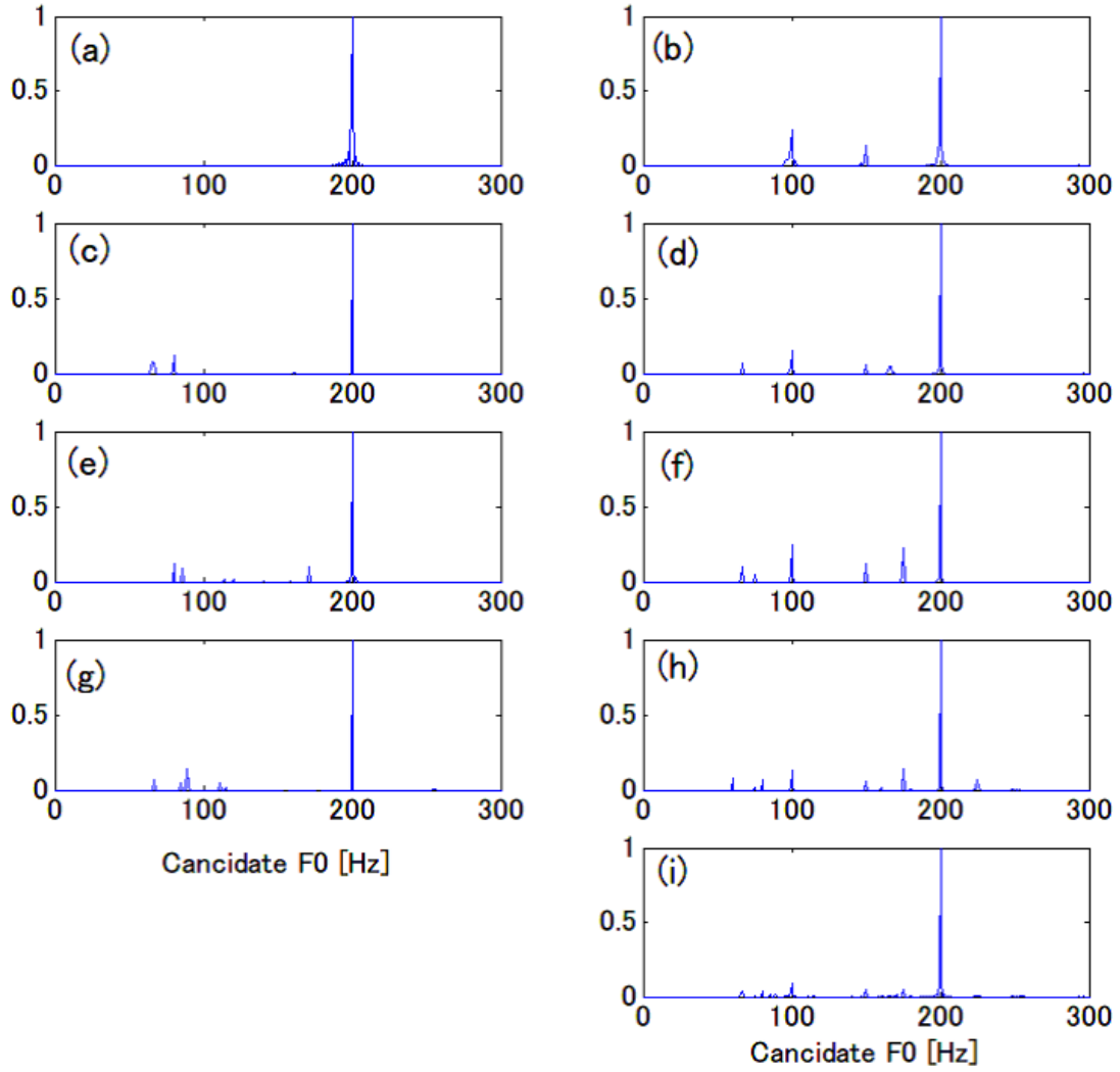
図 4.9: 総合評価指標の統合 : (a) 総合評価値 R_1 ( f_1, f_2, f_3 ), (b) 総合評価値 R_2 ( f_2, f_3, f_4 ), (c) 総合評価値 R_3 ( f_3, f_4, f_5 ), (d) 総合評価値 R_4 ( f_4, f_5, f_6 ), (e) 総合評価値 R_5 ( f_5, f_6, f_7 ), (f) 総合評価値 R_6 ( f_6, f_7, f_8 ), (g) 総合評価値 R_7 ( f_7, f_8, f_9 ), (h) 総合評価値 R_8 ( f_8, f_9, f_{10} ), (i) 最終総合評価値
