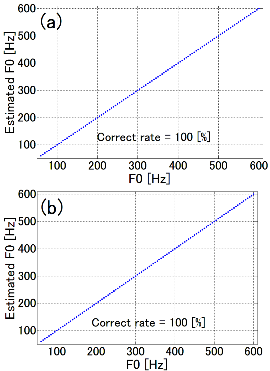
図 3.10: FreeDAM の動作検証 : (a) 1 次～3 次調波を利用した場合, (b) 4 次～6 次調波を利用した場合
