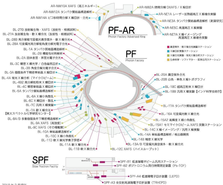
図 42 フォトンファクトリーにおけるビームラインマップ 出典：(KEK 2018)
