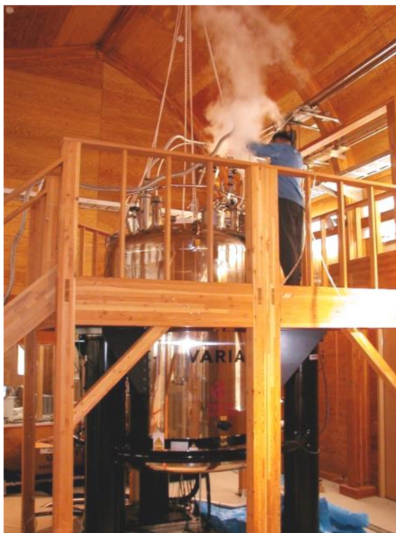
図 19 液体ヘリウムの充填作業 出典：(理化学研究所 NMR 施設 2018)
