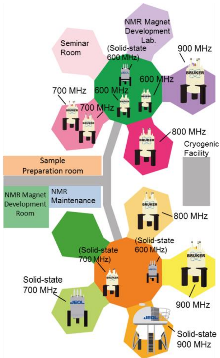
図 17 施設における NMR 配置図 出典：(理化学研究所 NMR 施設 2018)
