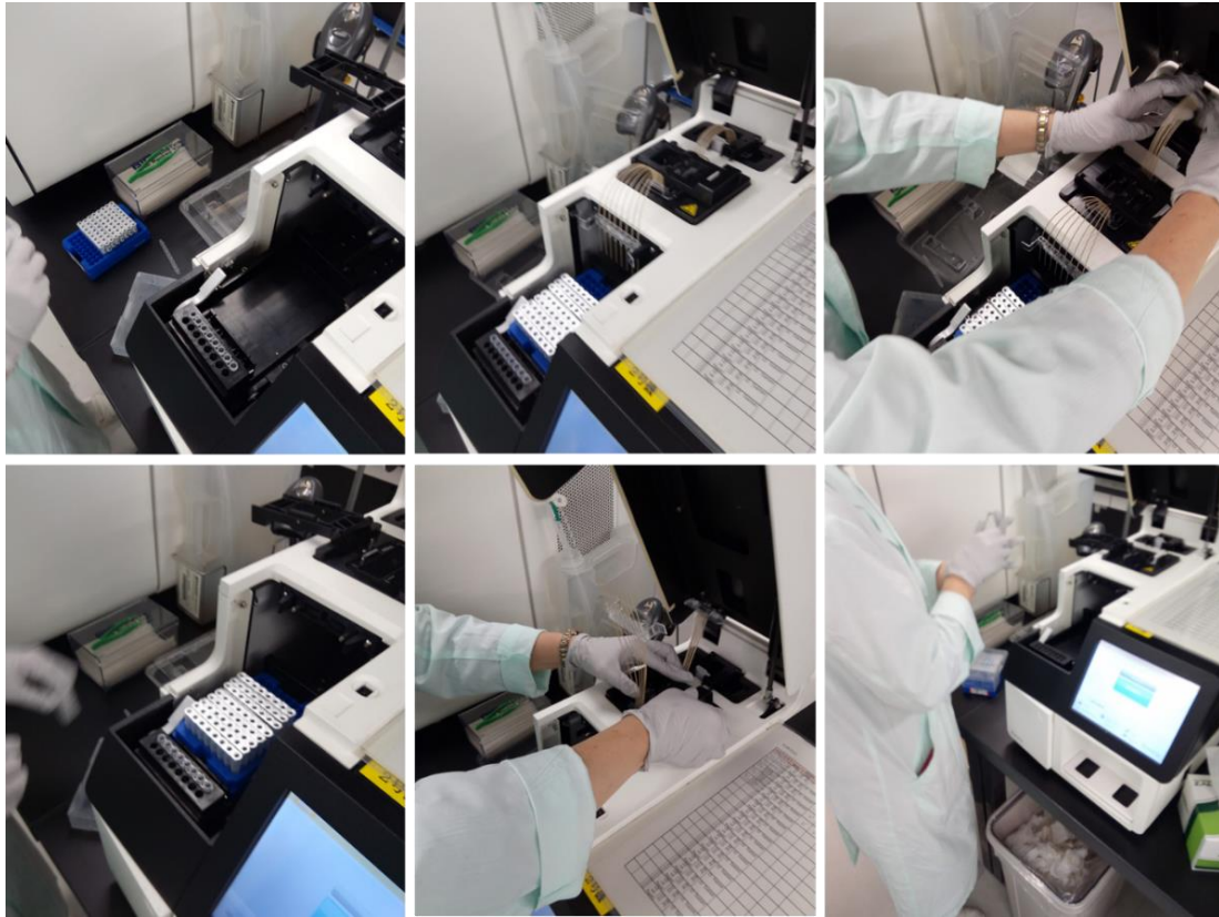
図 27 測定サンプルをシーケンサーに装てん 出典：筆者撮影（2018）
