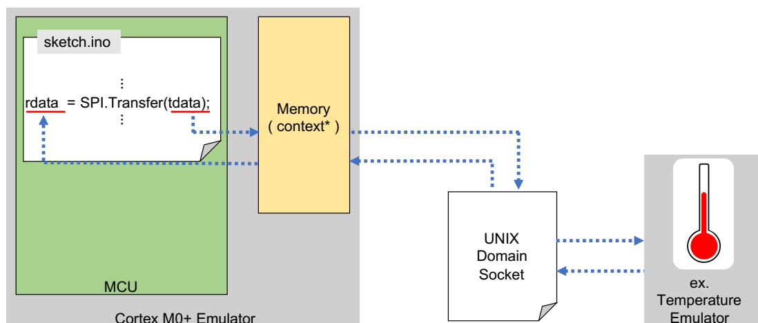
図 5.6: 疑似 SPI I/O モデル
