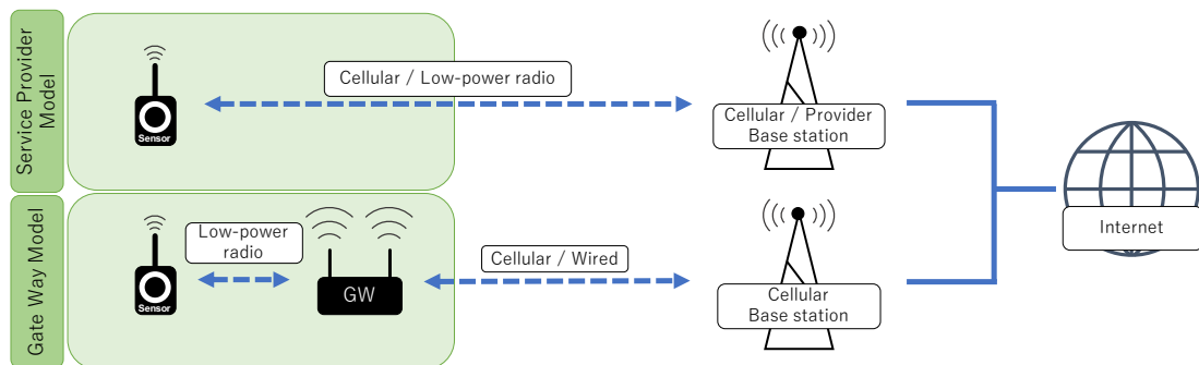
図 2.1: IoT のネットワーク接続モデル
