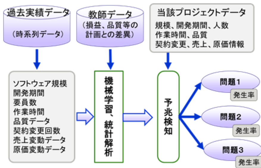
図 6-12 プロジェクトの状況悪化の予兆検知
