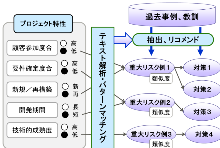
図 6-13 リスクの抽出と対策の助言
