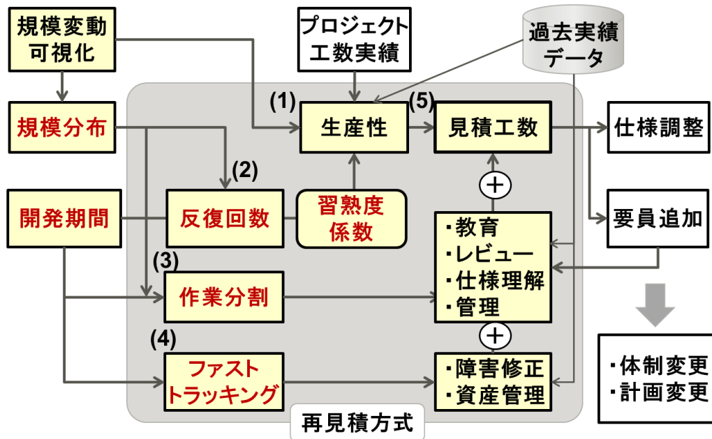
図 4-18 変動要因を考慮した工数の再見積方式（再掲）
