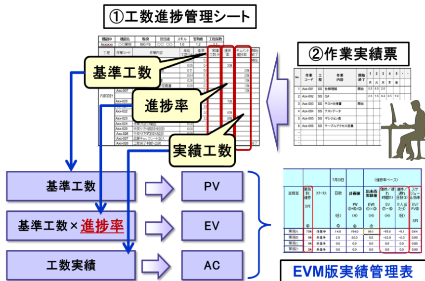
図 4-9 EMV の適用方法
