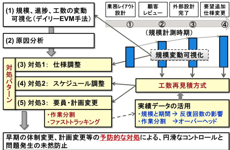
図 4-20 変動可視化によるコントロールのパターン
