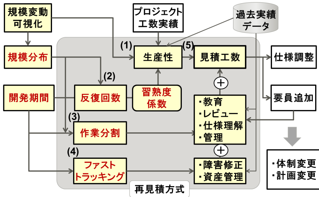
図 4-16 変動要因を考慮した工数の再見積り方式
