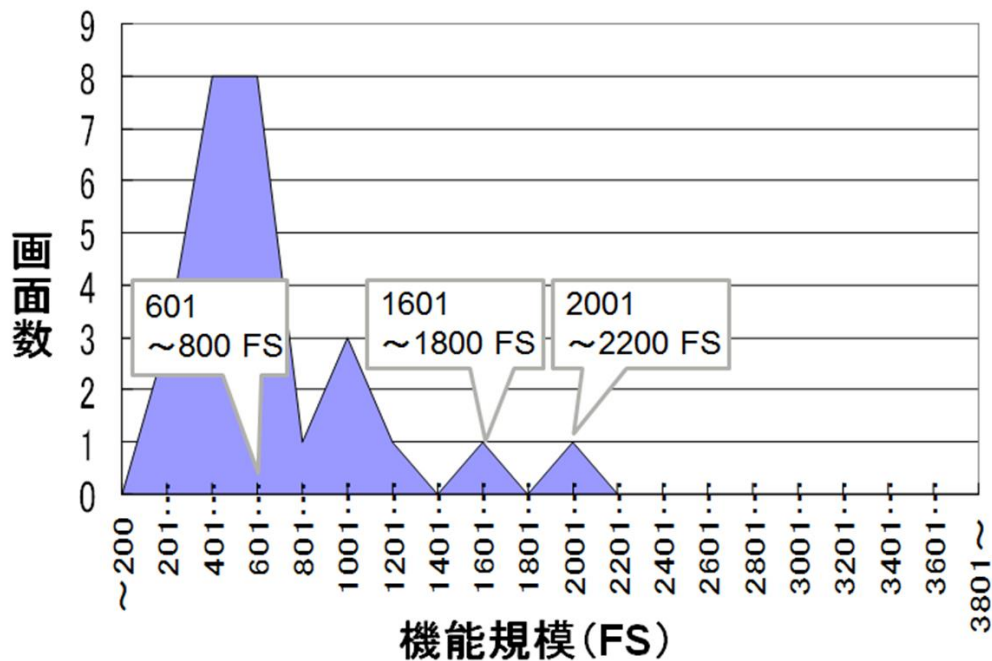
図 4-15 画面単位の規模分布図
