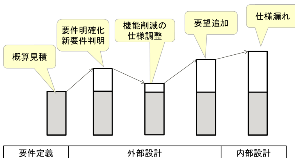
図 4-13 ソフトウェア規模の変動と対処の例
