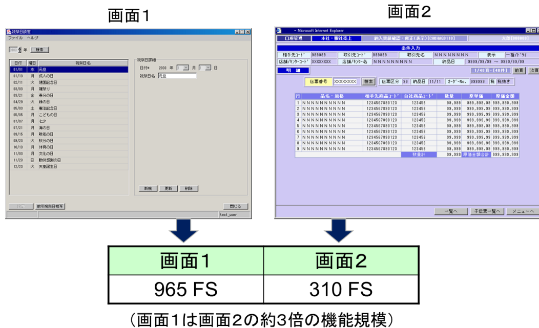
図 3-6 FS の計測事例の比較
