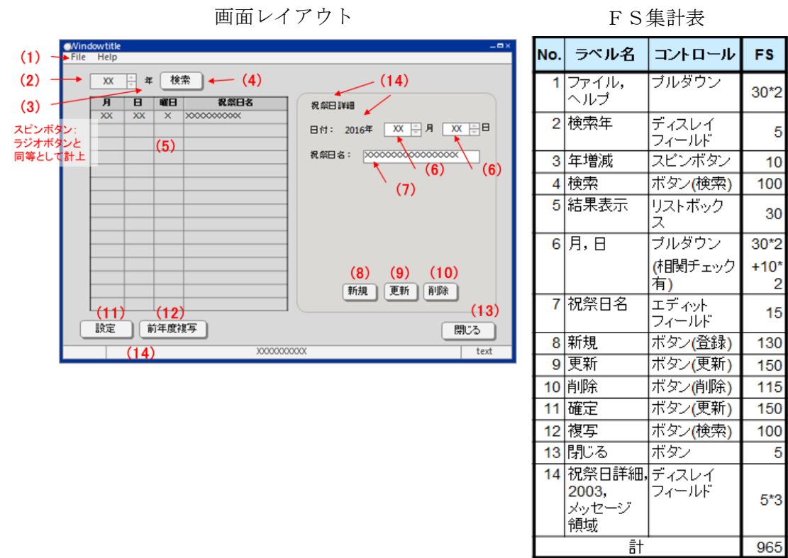
図 3-4 Web システムの画面レイアウトの例と FS 集計表
