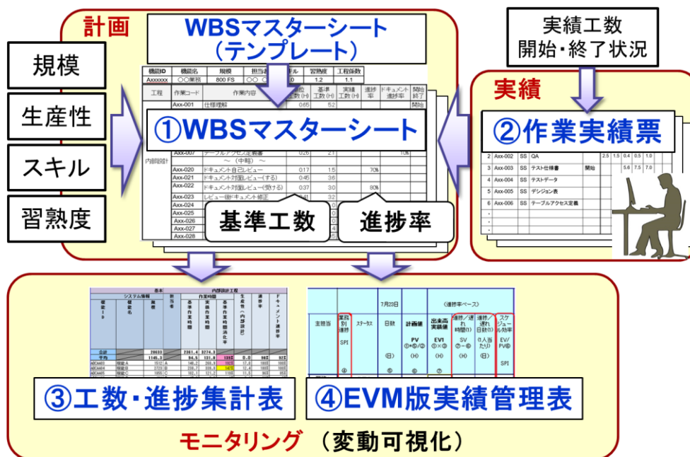
図 4-3 変動可視化手法「デイリーEVM 手法」の全体像
