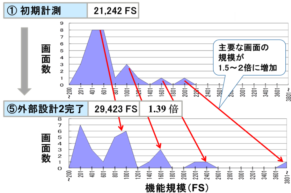
図 5-9 機能規模の変動結果
