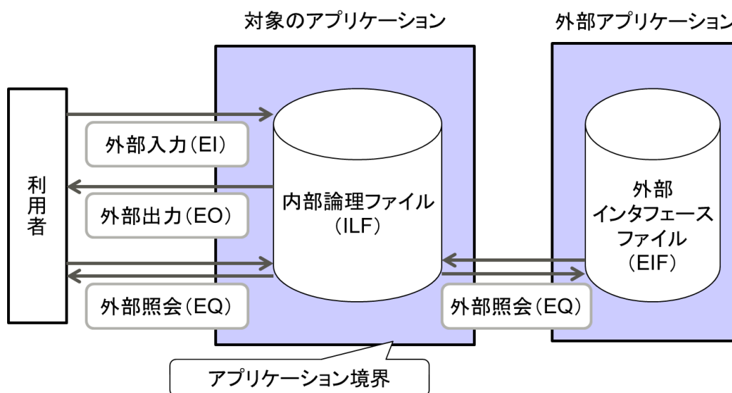
図 3-2 FP 法による計測対象としてのアプリケーションのモデル
