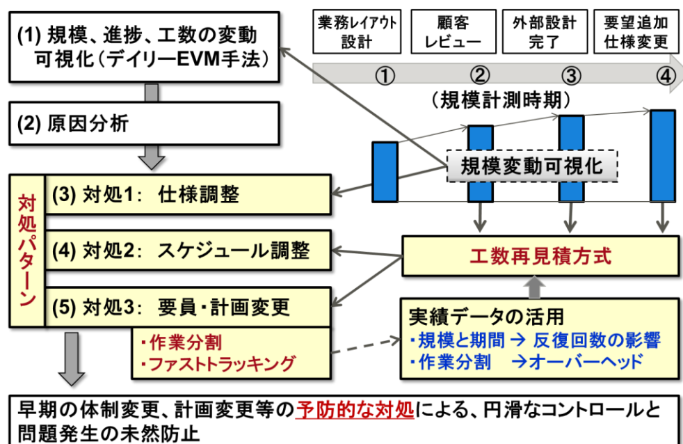
図 8-2 変動可視化によるコントロールプロセス（再掲）
