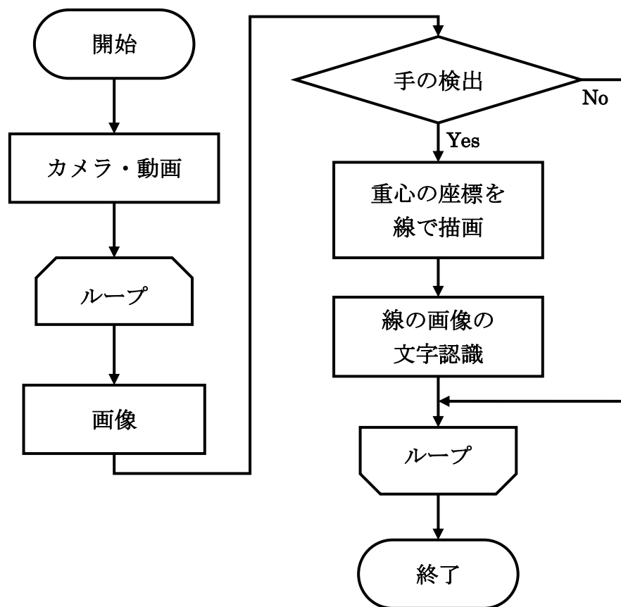
図 3.1 本研究のフローチャート
