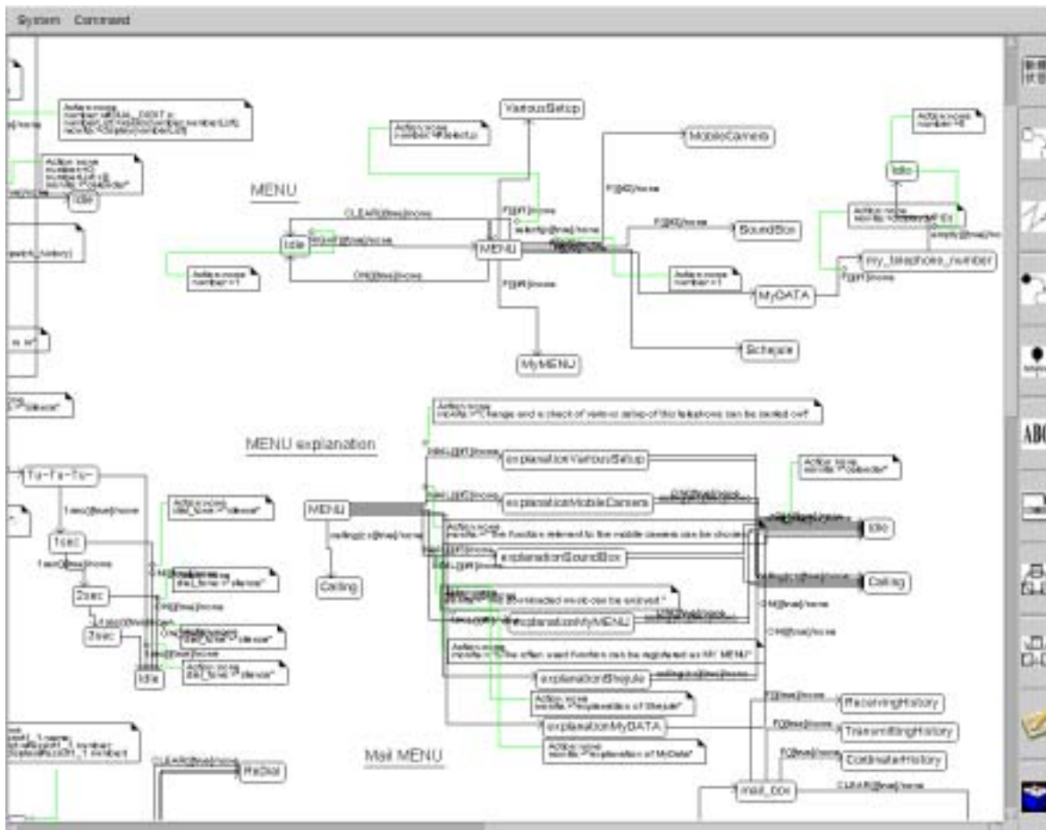
図 4.8: MobilePhone クラスの状態遷移図 4
