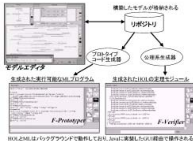
図 2.1: F-Developer
