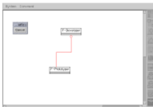
図 3.7: 集約作成
