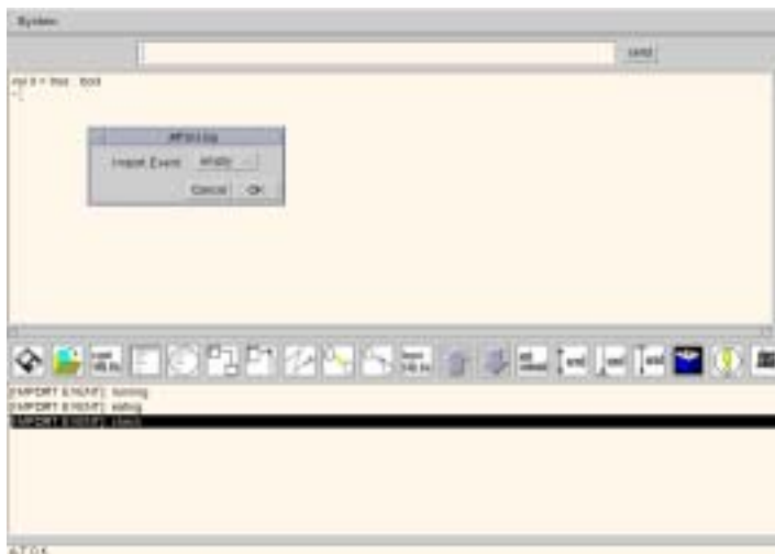
図 3.34: IMPORT EVENT
