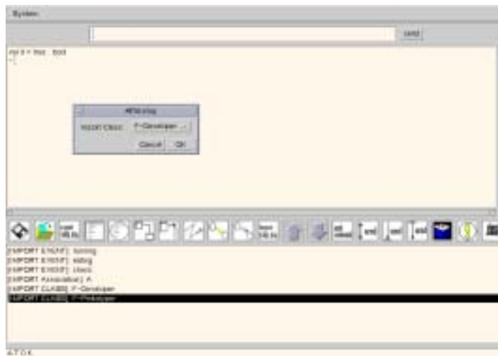
図 3.36: IMPORT CLASS
