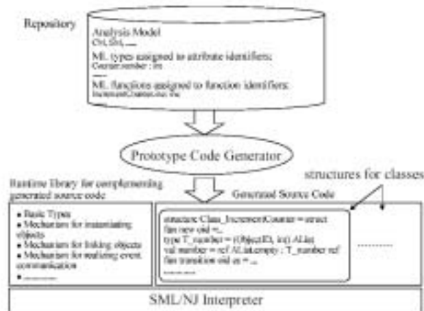
図 2.4: プロトタイプ実行の仕組み
