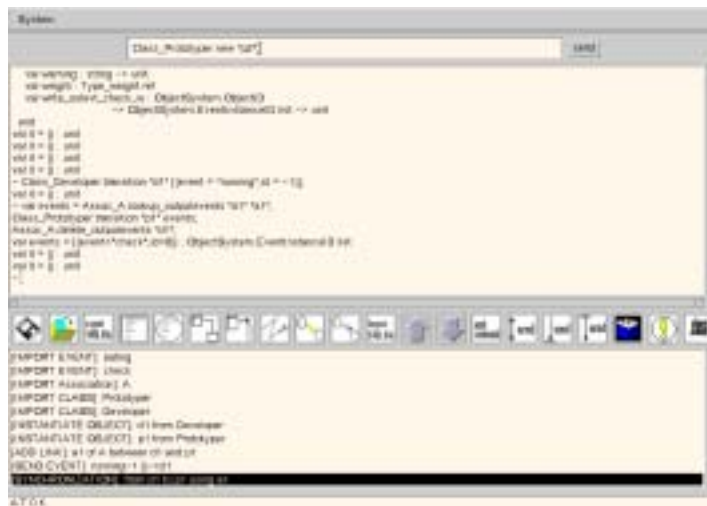
図 3.66: 開発者によるオブジェクト生成 2
