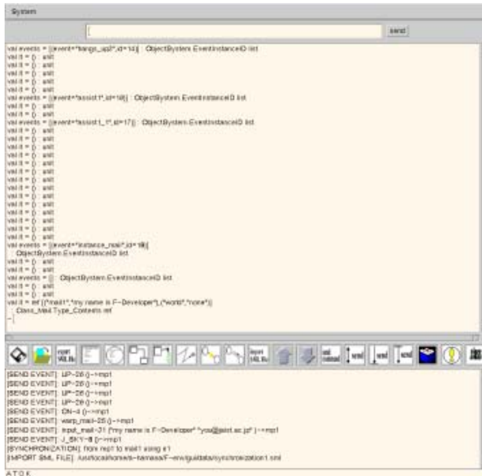
図 4.16: 携帯情報端末モデルのプロトタイプ実行の様子
