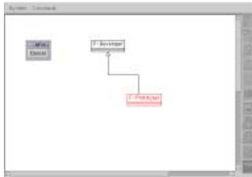
図 3.8: 汎化作成
