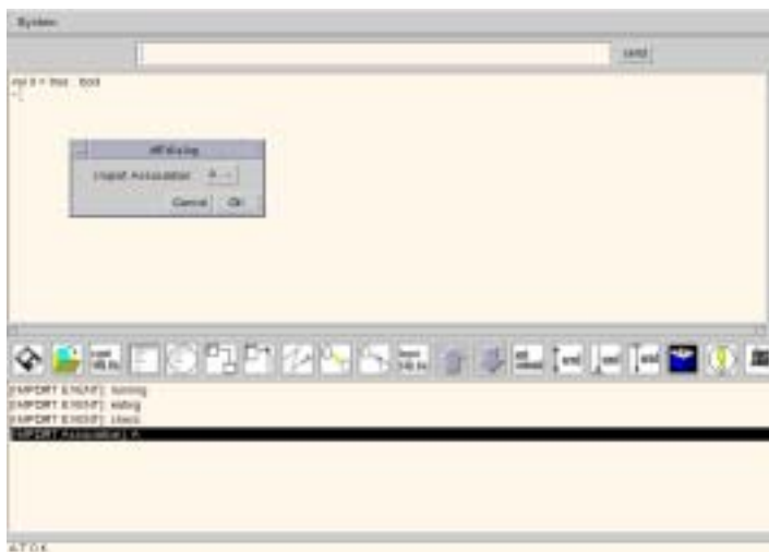
図 3.35: IMPORT Association
