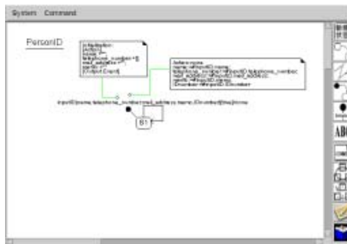
図 4.15: personID クラスの状態遷移図
