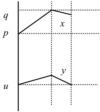
図 4.4: 例題のモデルのプロット
