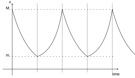
図 2.2: サーモスタットの振る舞い
