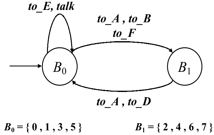
図 3.10: 図 3.3 の縮約エージェントネット
