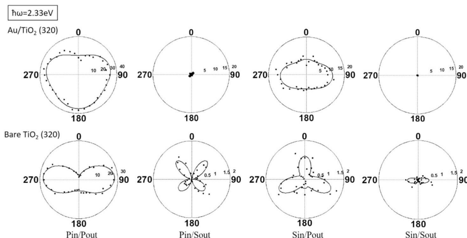
図 4 Au/TiO 2 (320)および TiO 2 (320)界面の方位角依存 SHG 強度パターン。励起光の光子エネルギーは 2.33eV である。ゼロ度は、入射面に [2\bar{3}0] 方向が含まれる配置に対応する。入射角は 45^\circ 。点と線がそれぞれ実験と計算。
