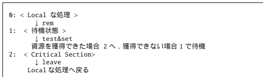
図 5.5: Test & Set に基づく相互排他システムの各プロセスの動作
