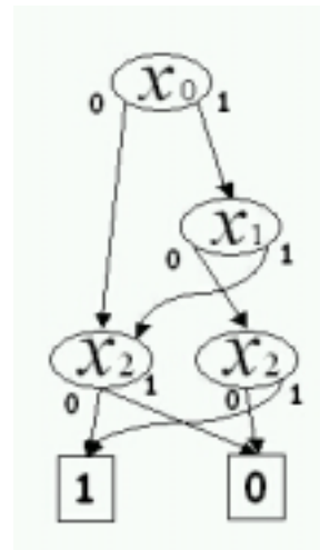
図 2.3: 論理式 P に対する決定木 (最適化後)
