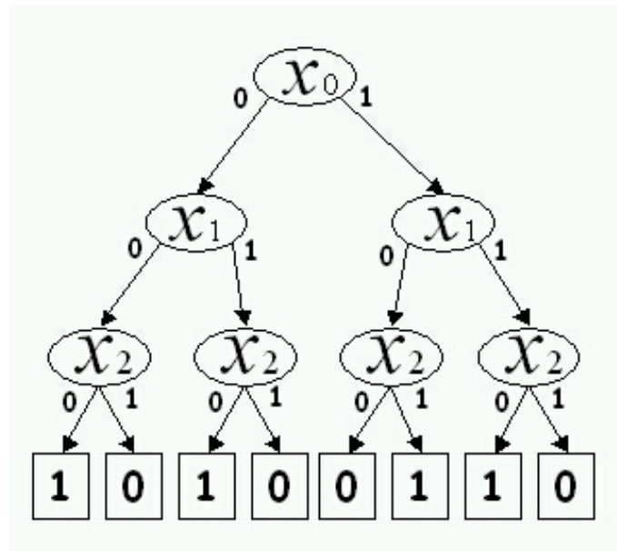
図 2.1: 論理式 P に対する決定木 (最適化無し)
