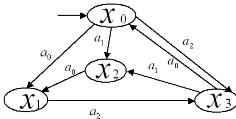
図 4.2: 有限化した振舞仕様の状態遷移
