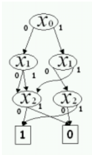
図 2.2: 論理式 P に対する決定木 (最適化途中)
