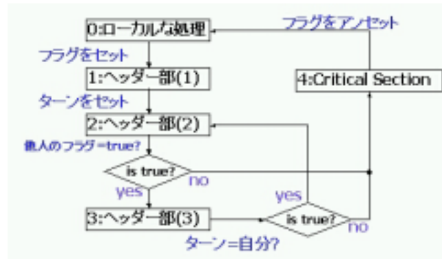
図 5.9: 各プロセスの動作
