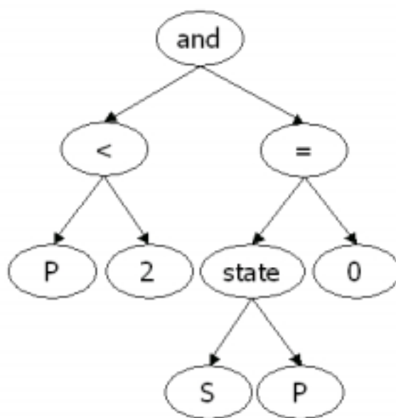
図 4.9: 等式 E の if 節の内部表現
