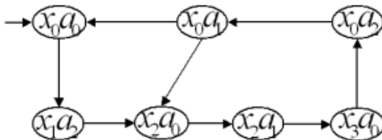
図 3.5: SMV 言語で扱う状態遷移機械の例
