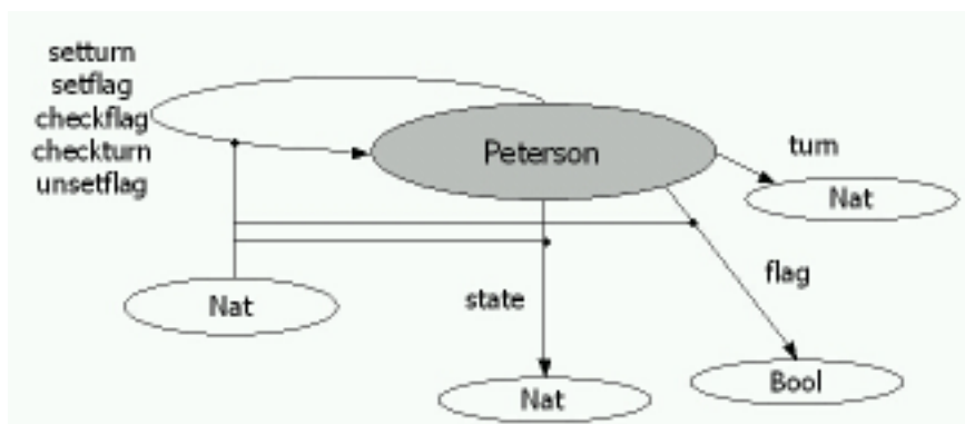
図 5.10: 振舞仕様による Peterson のアルゴリズムのモデル
