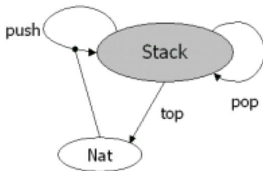
図 3.3: 自然数スタックの振舞仕様に対する ADJ 図
