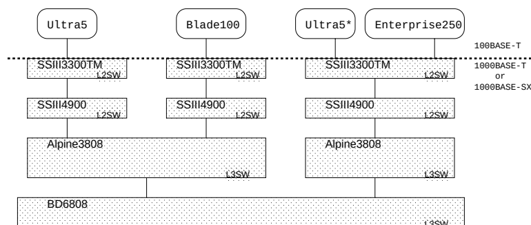
図 6.9: 実験環境ネットワーク概略図
