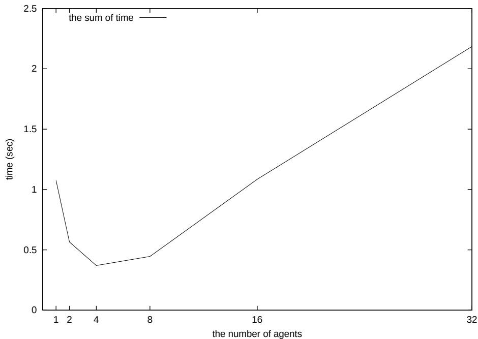
図 6.14: 32 台監視時のエージェント数による総時間変化
