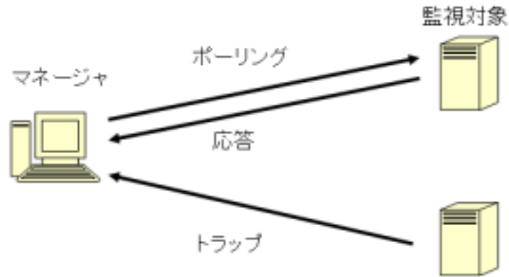
図 3.1: SNMP 方式の概観図
