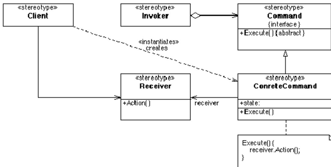
図 2.6: Command パターン
