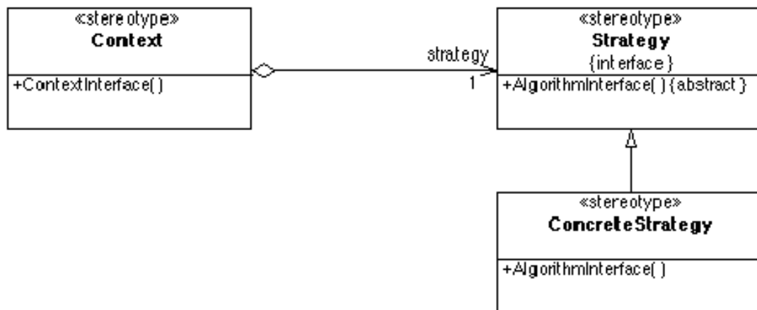
図 2.5: Strategy パターン
