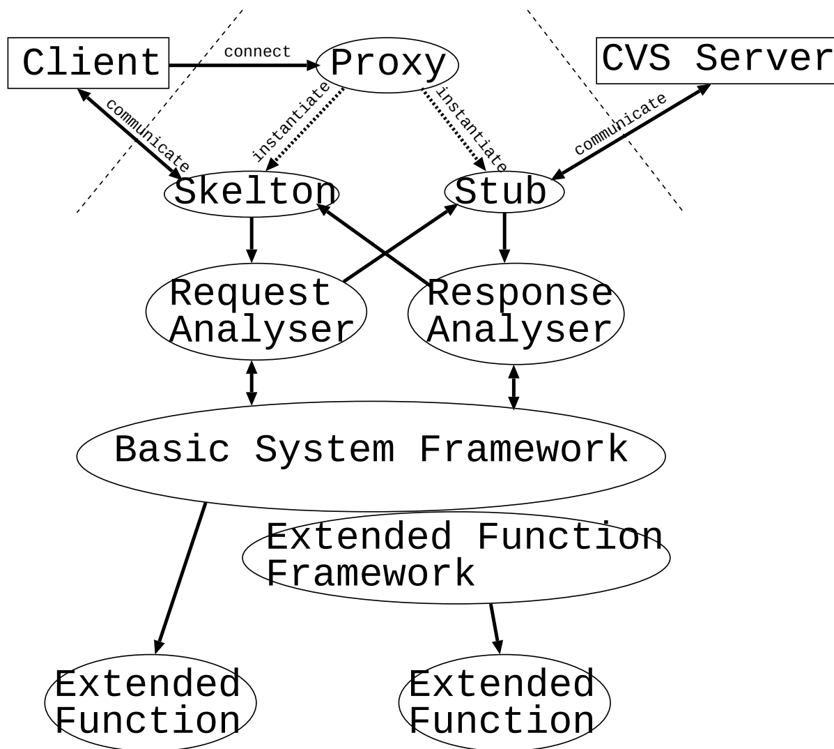
図 4.2: オブジェクトを用いたプロトタイプシステムの設計 (概念図)
