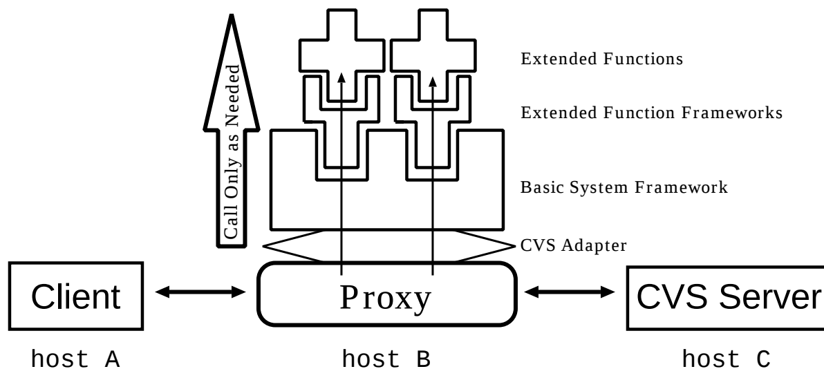
図 4.1: プロトタイプシステムの実装アーキテクチャ
