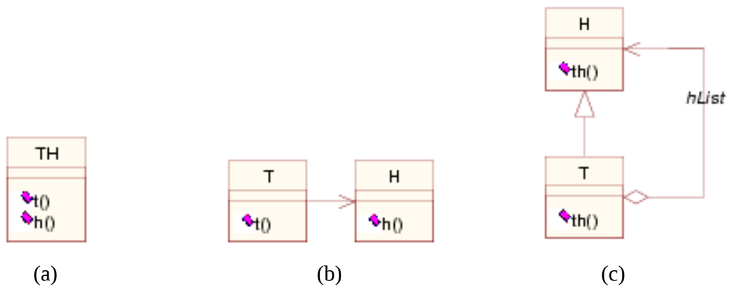
図 2.7: Unification メタパターン (a), 1:1 Connection メタパターン (b), 1:N Recursive Connection メタパターン (c)
