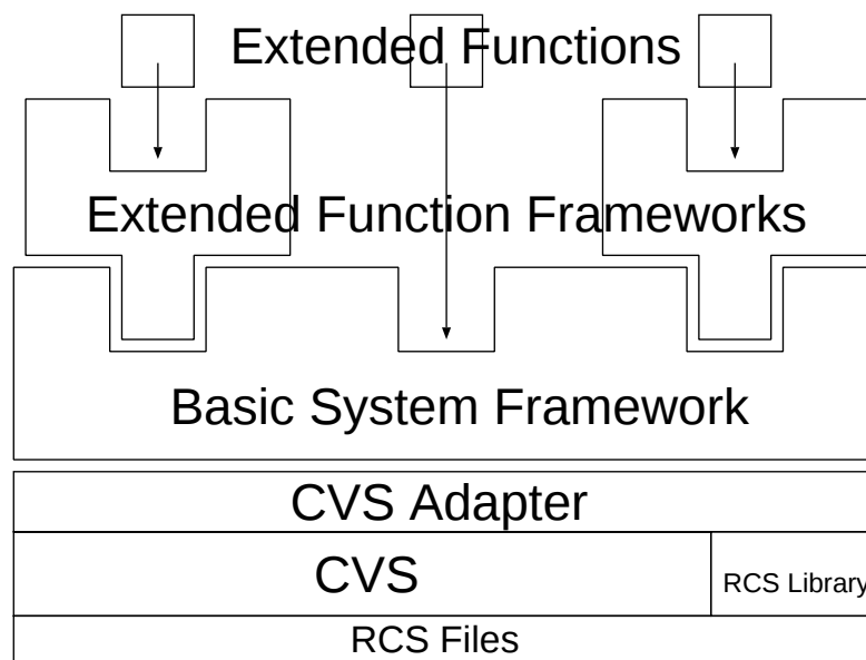
図 3.1: 6 層レイヤアーキテクチャ
