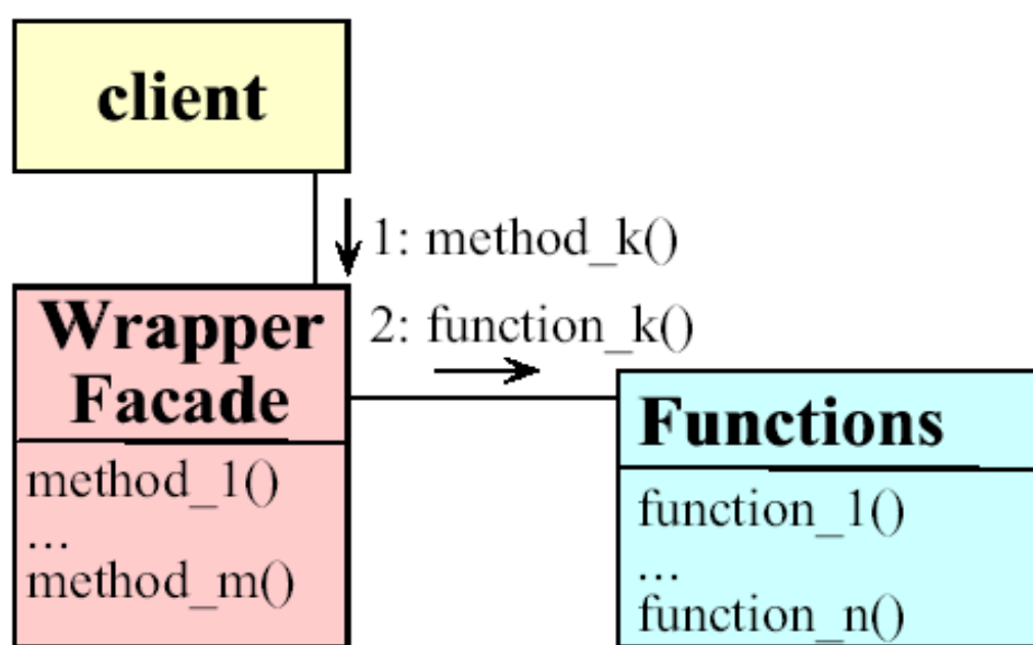
図 3.2: Wrapper Facade パターン
