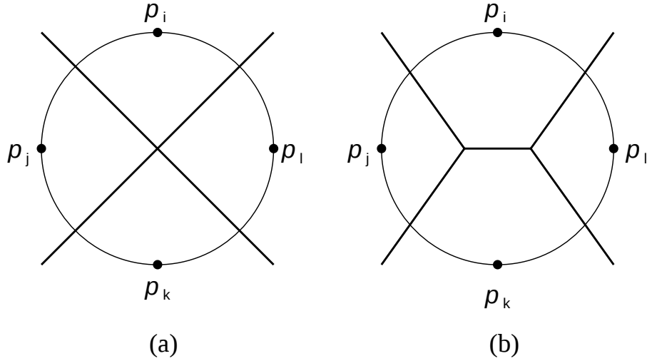
図 1.1: 縮退による位相矛盾: (a) 正しいボロノイ図, (b) 縮退により隣接関係が変わってしまう例.
