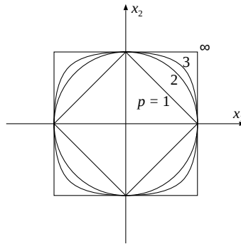
図 5.1: 1,2,3, \infty に関するミンコフスキー距離の等距離線
