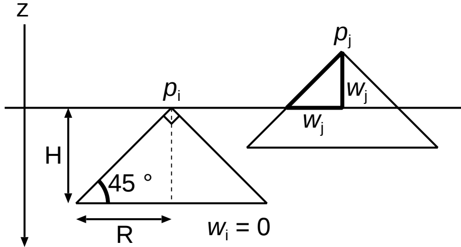
図 5.6: 加法重み付きボロノイ図に対する 3 次元距離関数
