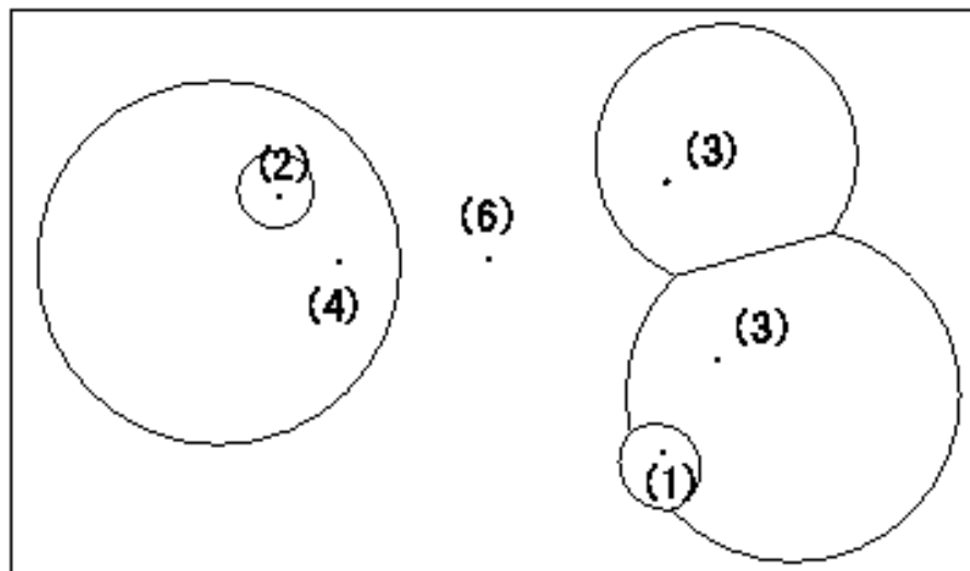
図 6.1: 乗法重み付きボロノイ図
