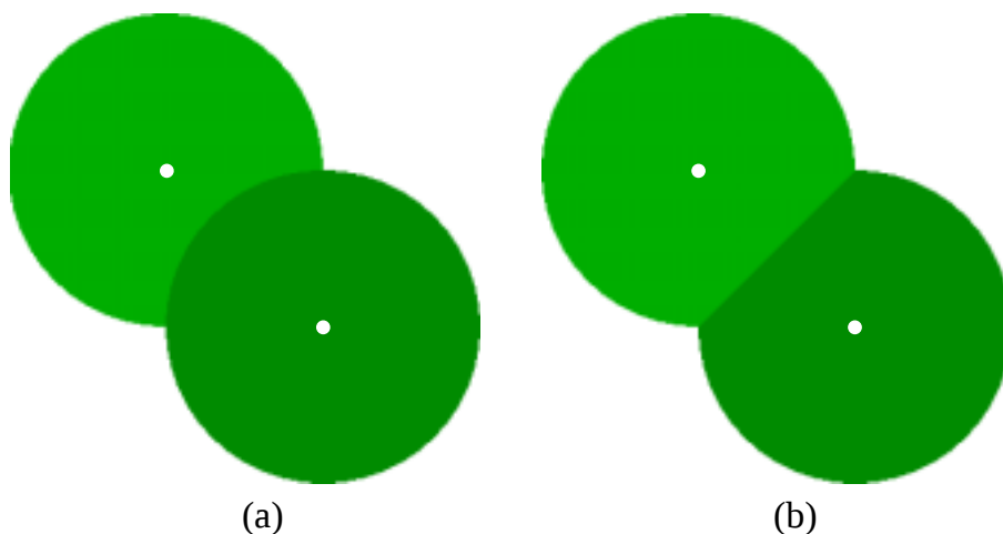
図 3.2: 隠面除去によるボロノイ領域の表現
