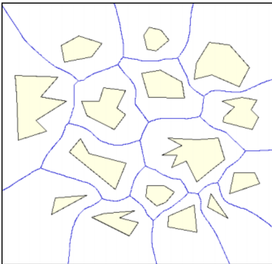
図 2.8: 多角形のボロノイ図
