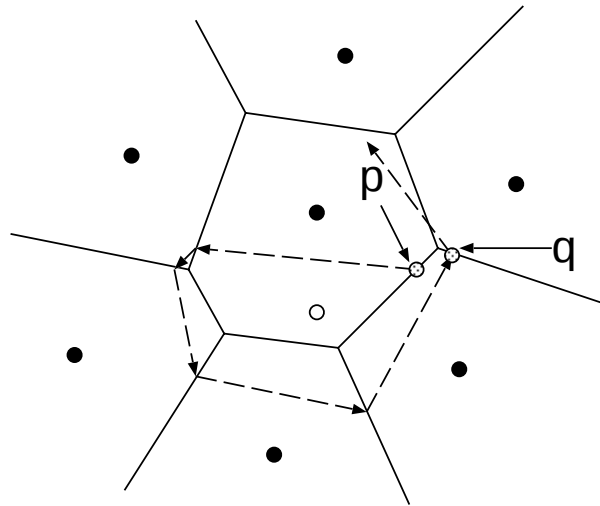
図 1.2: 数値誤差により閉じていない境界を出力してしまう例
