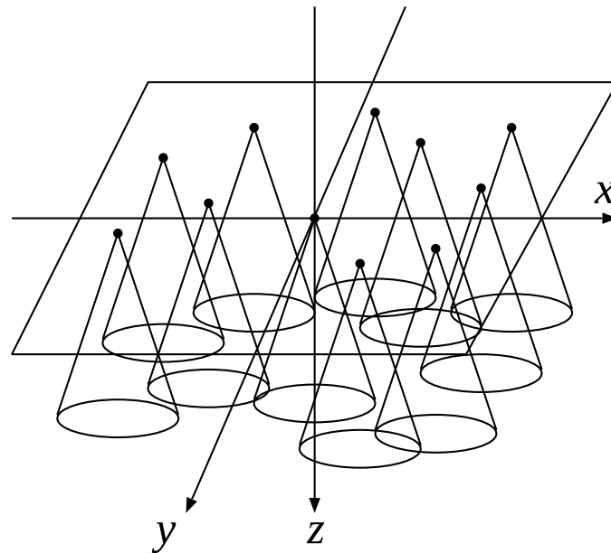
図 3.1: 点サイトのボロノイ図
