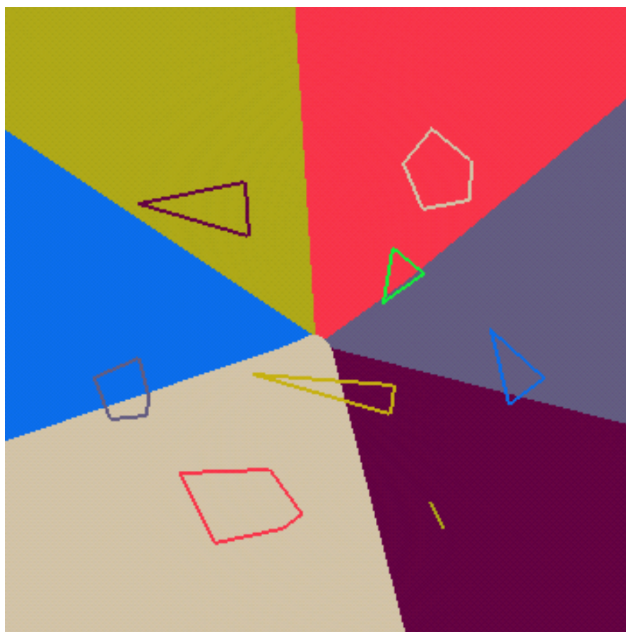
図 5.8: Hausdorff 距離のボロノイ図の例
