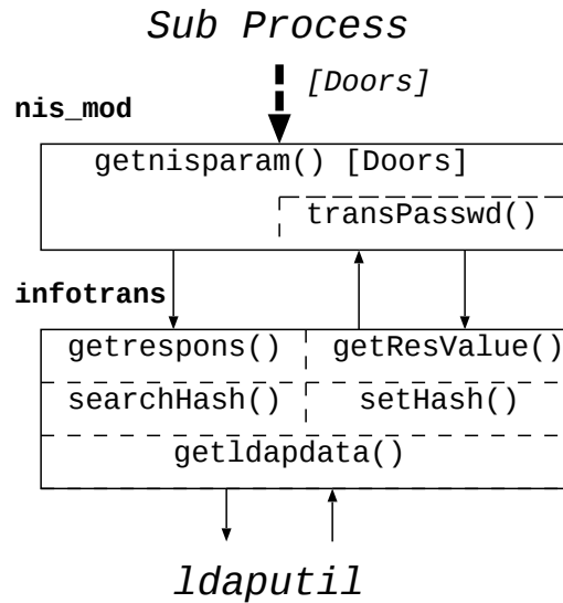
図 4.5: Data Transform Module
