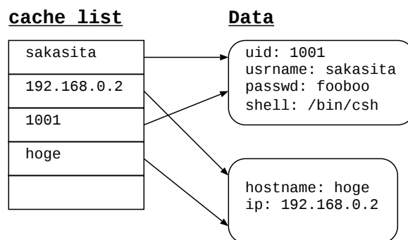
図 3.7: キャッシュリストとデータ
