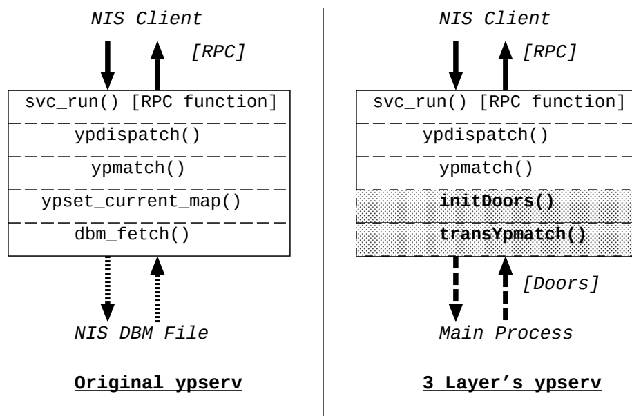
図 4.4: Request Server Module
