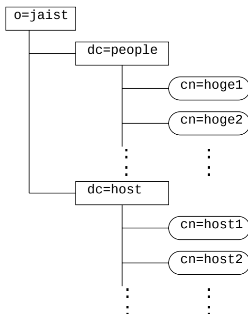
図 4.10: ツリー構成
