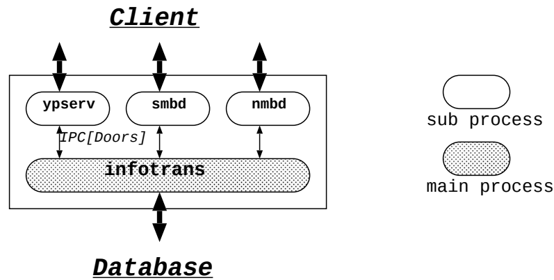
図 4.3: Naming Server Layer のプロセス
