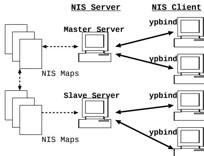
図 2.1: NIS 構成
