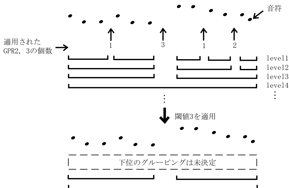
図 3.10 GPR4 のアプローチ
