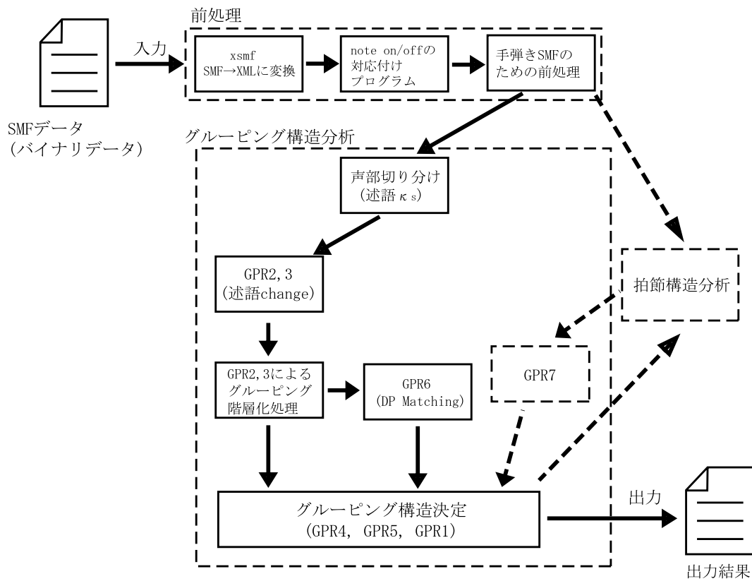
図 5.3 課題となるグルーピング構造分析システム
