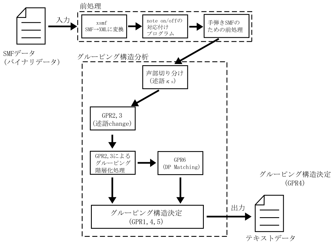
図 4.1 システム概要図
