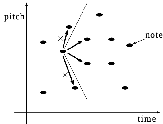
図 4.6 楔形の選択範囲の適用
