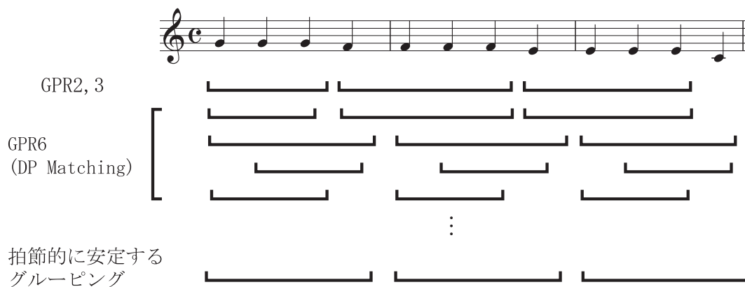
図 5.1 拍節構造分析の必要性
