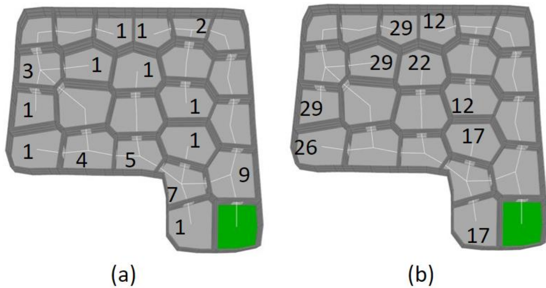
図 31: スタートから行き止まりまでの到達しにくさの計算手順. 緑の部屋がスタート地点. (a)割り当てられた次数(b) (a)で割り当てられた次数から計算された到達しにくさ
