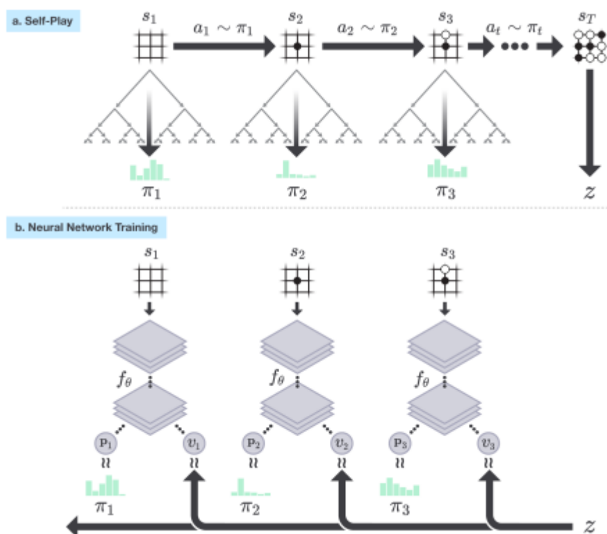
図 2.10 : AlphaGo Zero のニューラルネットワークの学習
