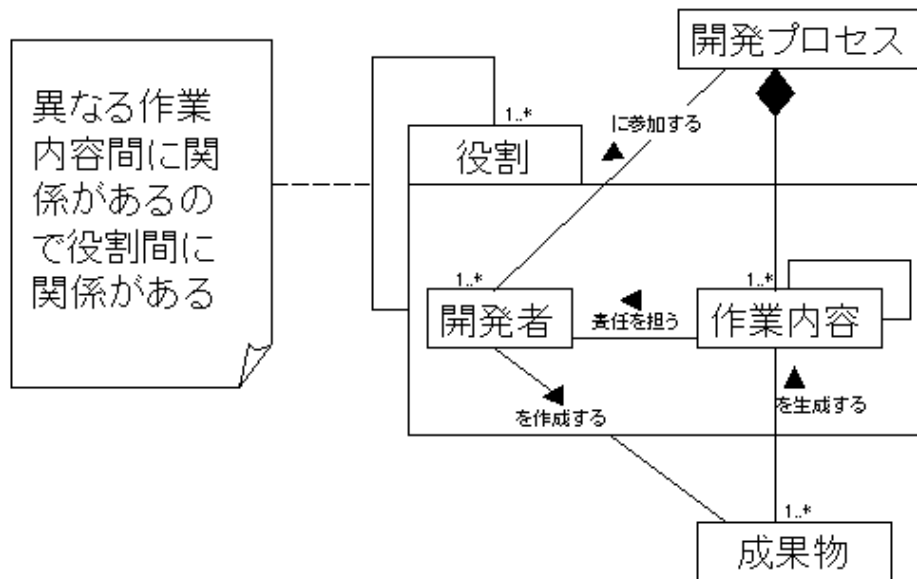
図 2.2: RUP の役割のメタモデル
