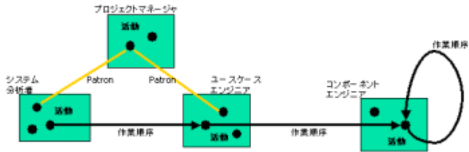
図 3.2: パトロン 作業の流れとは独立したコミュニケーションを示せる。
