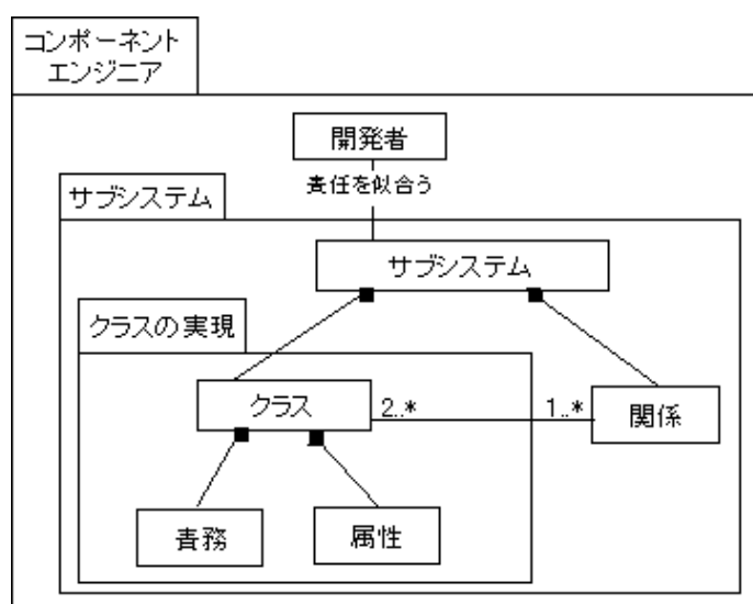
図 2.8: コンポーネントエンジニア
