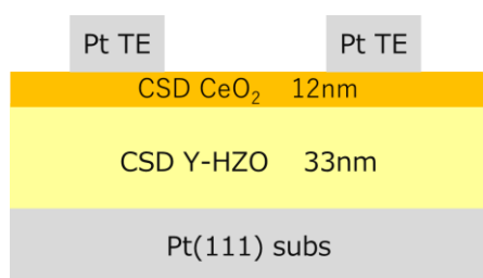
図 1. 試料構造
