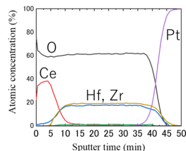
図 3. XPS による各元素の深さ方向分布
