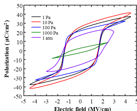
図 1.HZO 薄膜の P-E 測定結果
