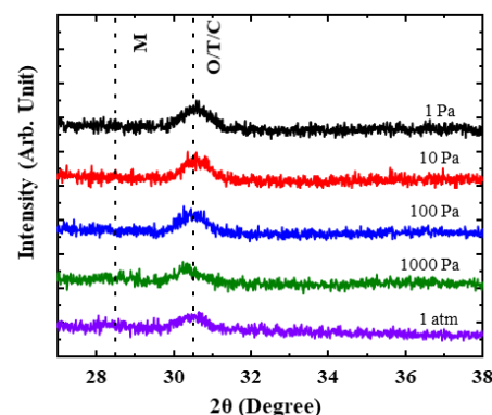
図 2. HZO 薄膜の XRD 測定結果
