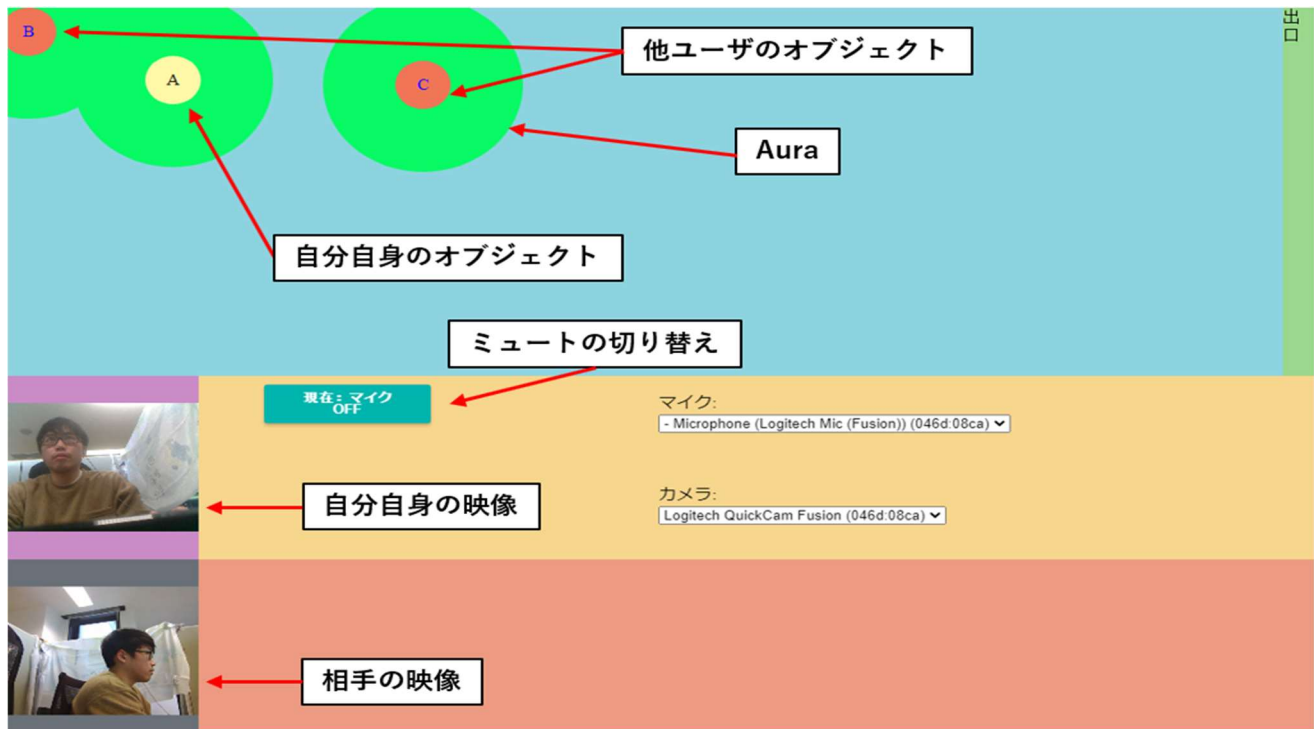
図 1 Commidor のユーザインタフェース
