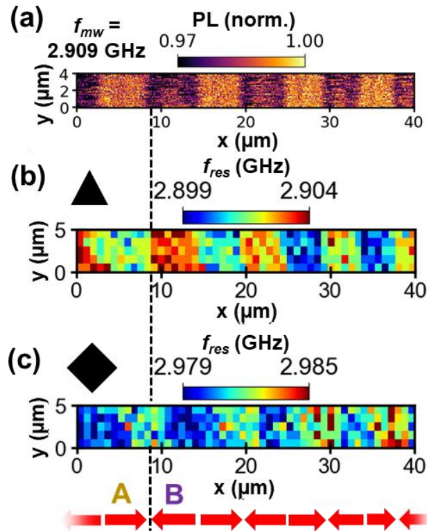
図 4.2.3: 磁気テープ上の Grid 計測の結果
