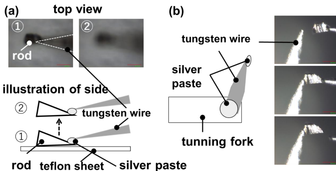
図 S3: ダイヤモンドロッドのタングステンワイヤへの取り付け方
