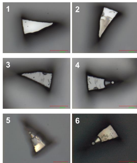
図 5.2.1: PVA および白金パラジウムのダイヤモンドロッドへのコーティングから除去までのプロセス: 1.ダイヤモンド表面の洗浄 2.PVA によるダイヤモンドの固定 3.白金パラジウムの蒸着 4.FIB 加工 5.王水による白金パラジウムの除去: 写真は王水中 6.PVA 除去後のダイヤモンドプローブ
