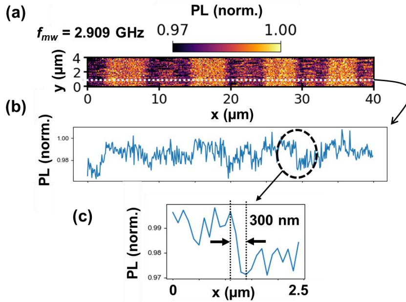
図 4.3.2: 空間分解能の見積もり
