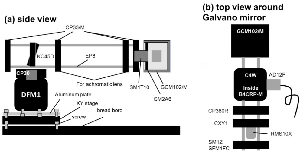
図 S8.2: 光学素子固定用部品の概要図 (a)側面および(b)上面図
