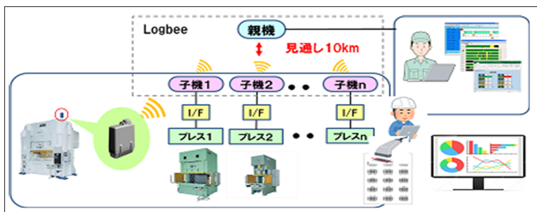
図 5. Haruca Smart Press 概要
