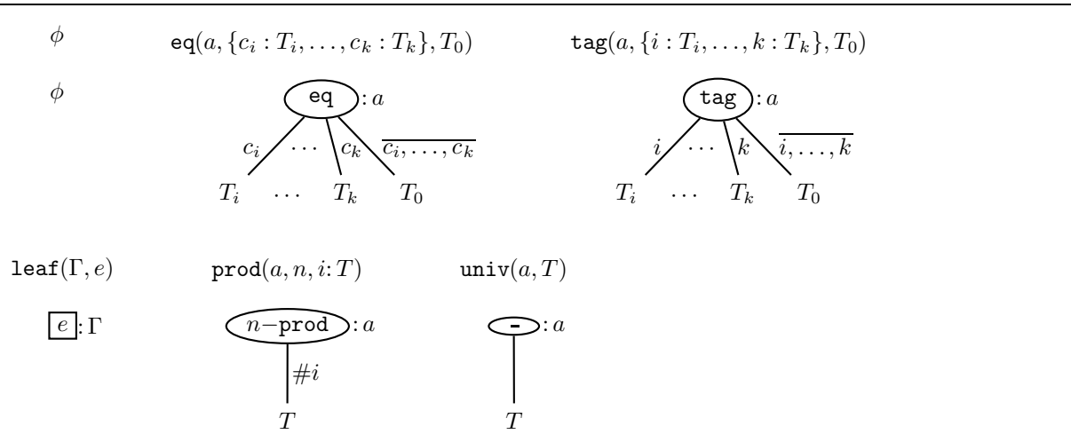
図 4.2: 決定木とその項表現の対応
