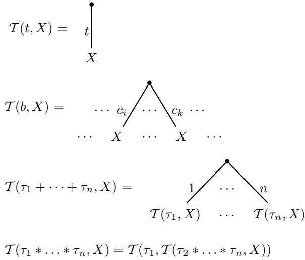
図 3.1: 型 \tau に属する項の全集合の木表現
