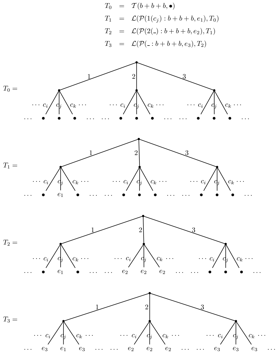
図 3.4: ラベル付けの例
