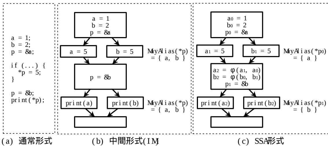
図 5.2: SSA 形式に対するフロー非依存のポインタ解析の例
