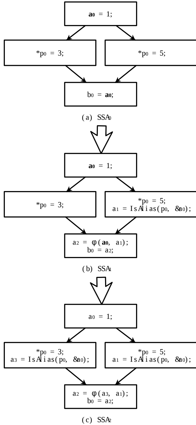
図 4.1: IsAlias 関数の挿入の例
