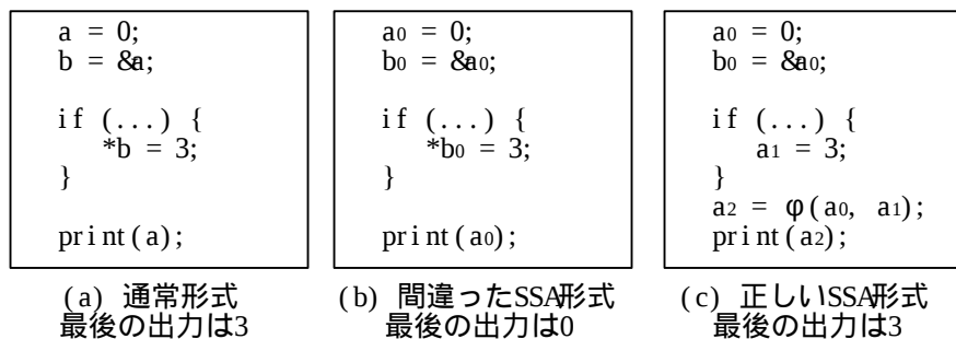
図 3.7: SSA 変換時のポインタの問題 1
