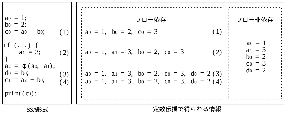
図 2.7: SSA 形式における定数伝播
