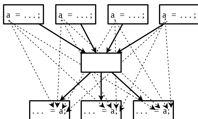
図 2.3: 使用と定義のリンク
