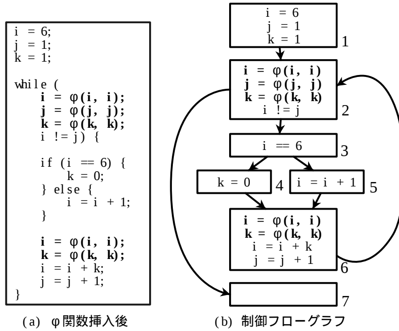
図 3.3: \phi 関数挿入後のプログラム
