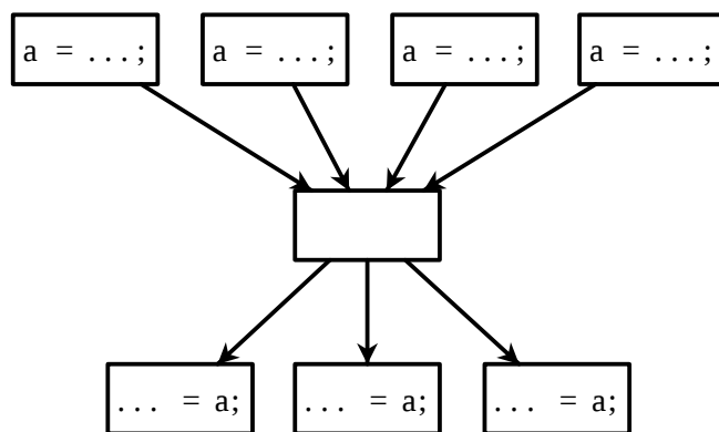
図 2.2: 分岐と合流のあるプログラム
