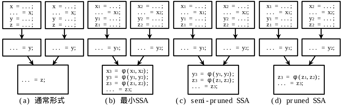
図 7.1: 3 種類の SSA 形式の違い
