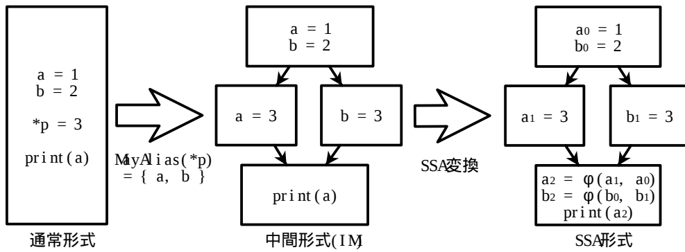
(a) ポインタ参照による定義を分岐に置き換える
