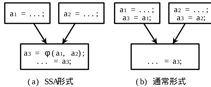
図 3.5: 単純な方法による SSA 逆変換
