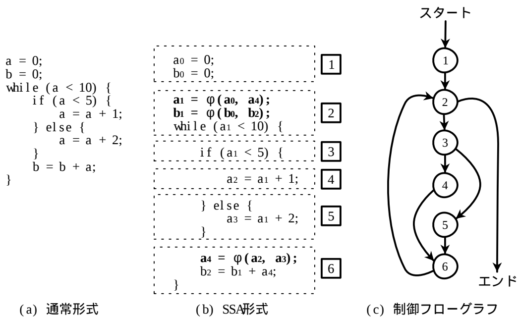
図 2.5: SSA 形式の例
