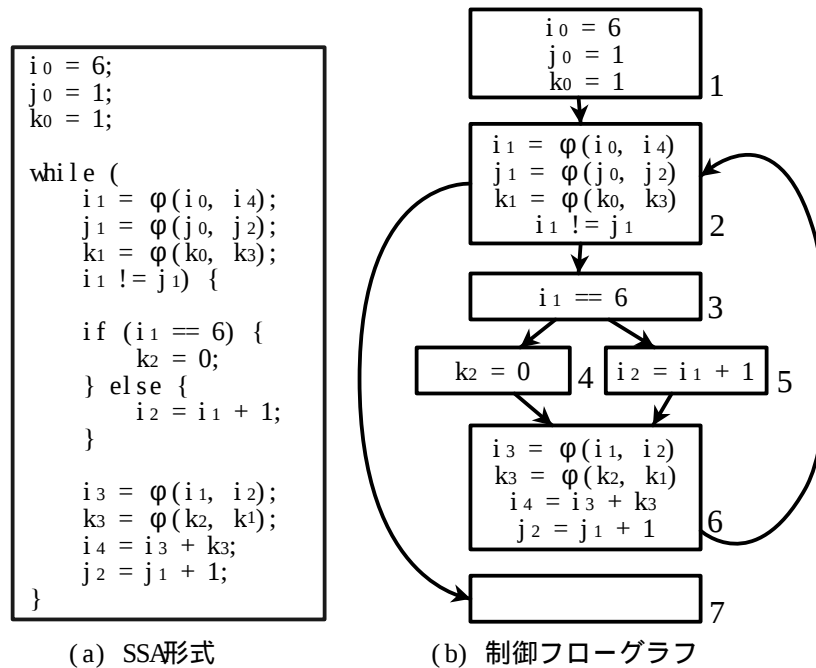
図 3.4: 変数名の付け替え後のプログラム
