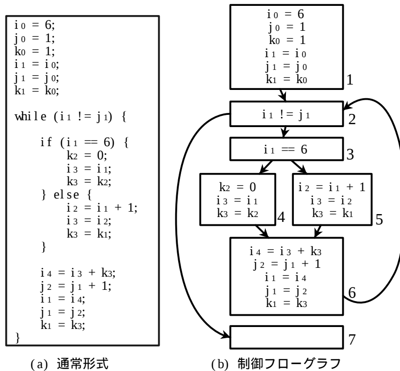
図 3.6: SSA 逆変換後のプログラム
