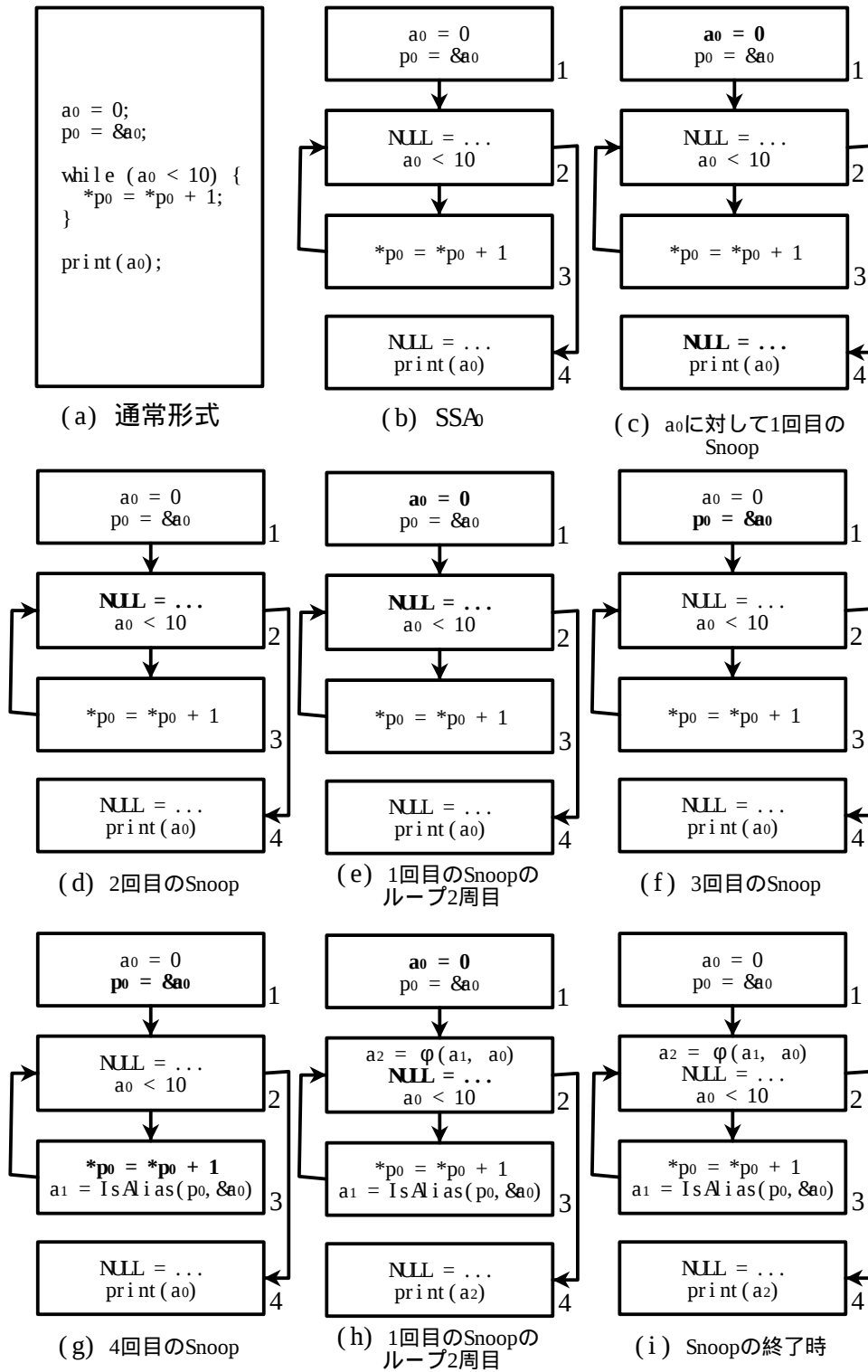
図 4.2: Cytron らのアルゴリズムの例
