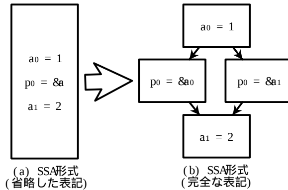
図 5.3: アドレス演算を分岐で表現する例
