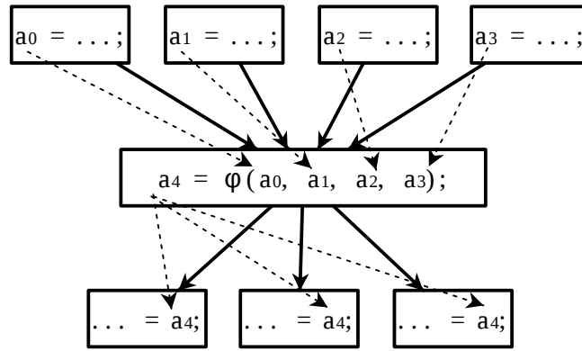
図 2.4: SSA 形式による使用と定義のリンク
