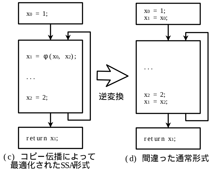
図 7.2: 単純な SSA 逆変換が上手くいかない例
