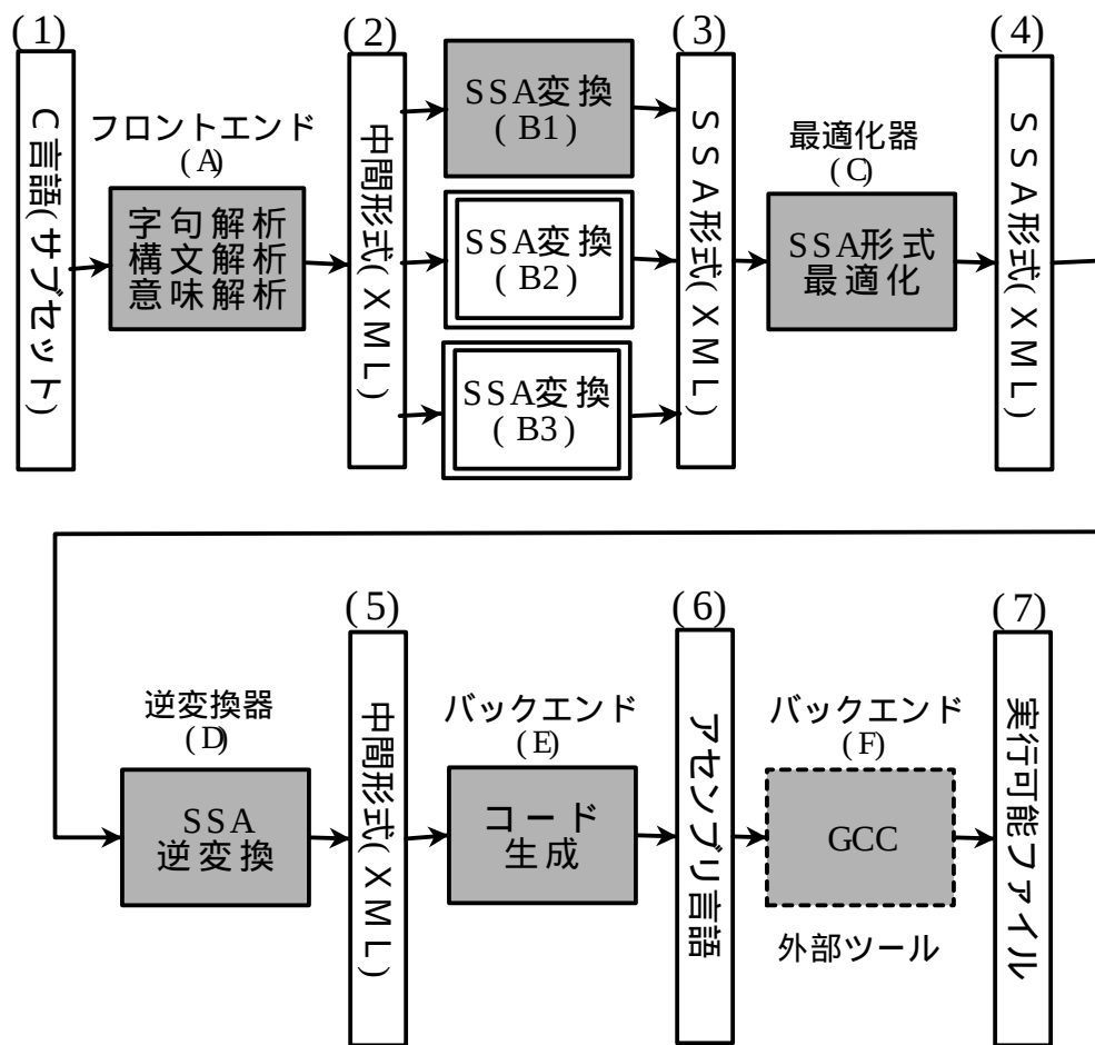
図 1.1: 評価環境の全体図
