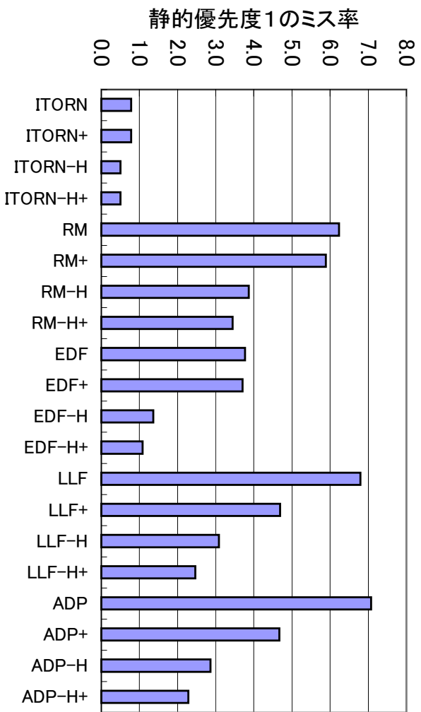
図 4.3: 静的優先度1のタスクにおける平均ミス率.
