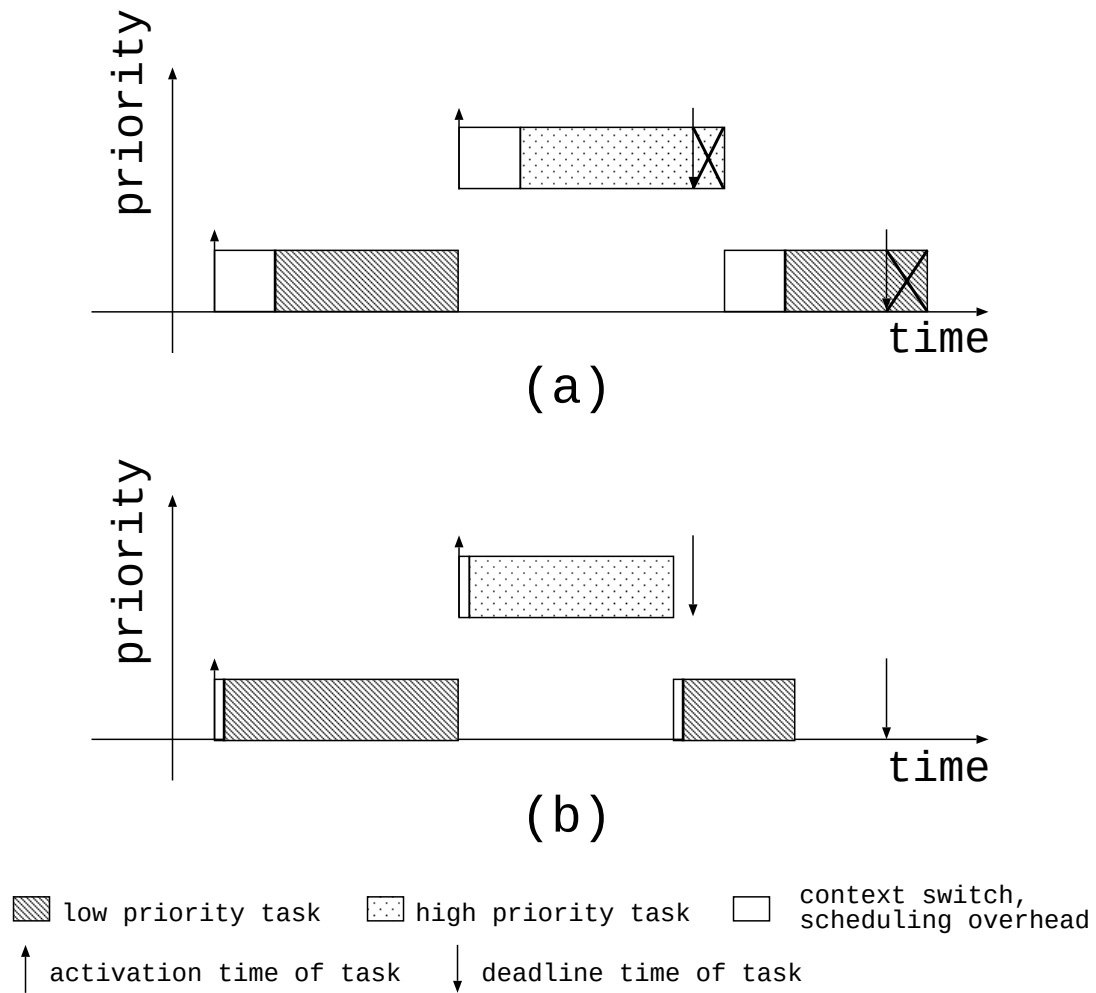
図 3.1: オーバヘッド軽減によるデッドラインミス削減例.
