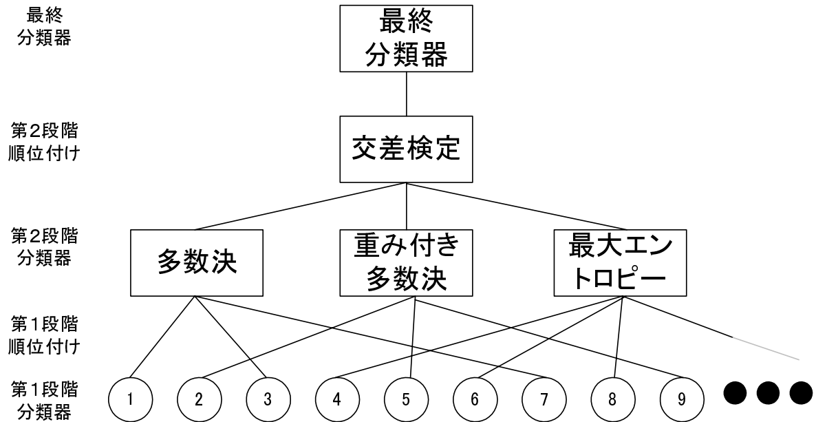
図 2.1: Klein の方法
