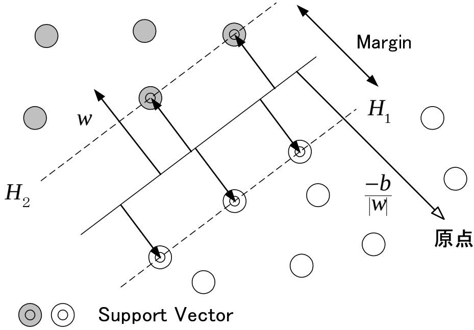
図 3.1: SVM 概要
