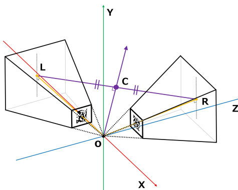
図 11 2つの AR マーカからなる中央方向視点の求め方
