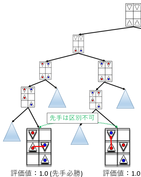
図 6 CFR-B が上手いかわかないケース
