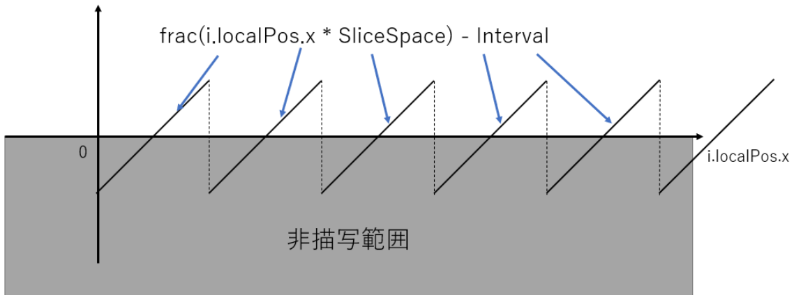
図 3.6: 表示・非表示を判定する \text{clip}(\text{frac}(i.\text{localPos}.x * \text{SliceSpace}) - \text{Interval}) のグラフ
